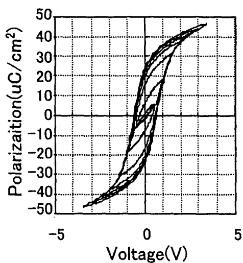
FIG. 5C 25nm
