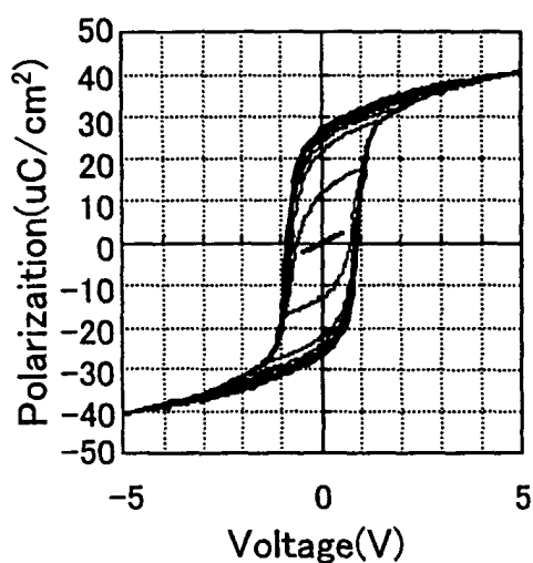
FIG. 5A 100nm
