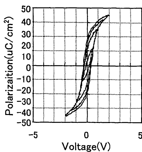
FIG. 5D 15nm
