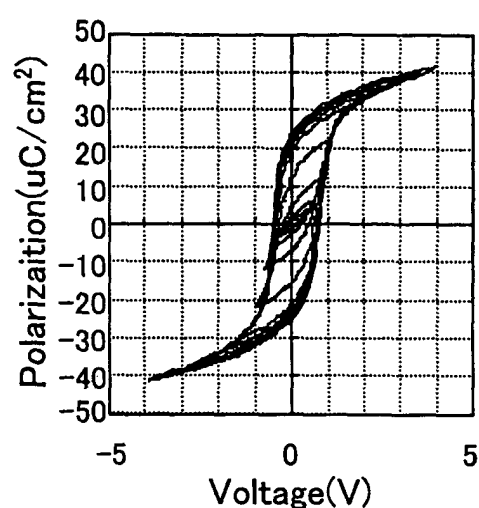
FIG. 5B 80nm
