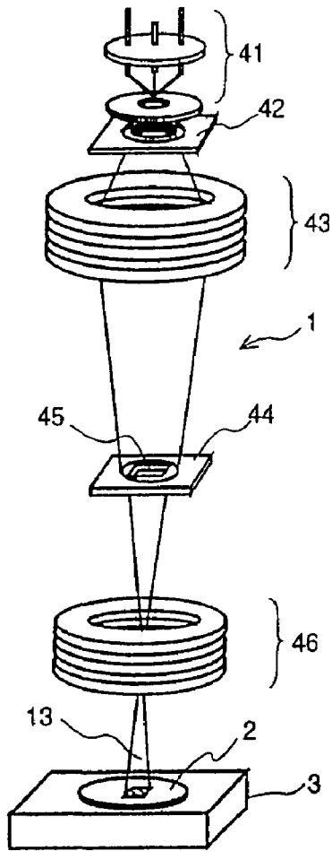
FIG. 5 A
