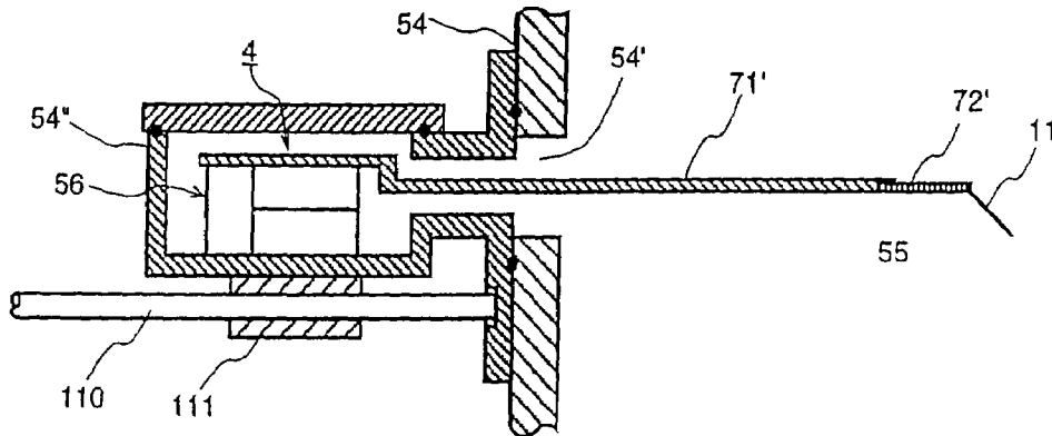
FIG.20C
