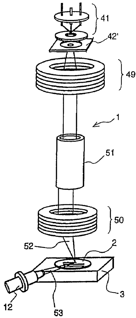
FIG. 5 C
