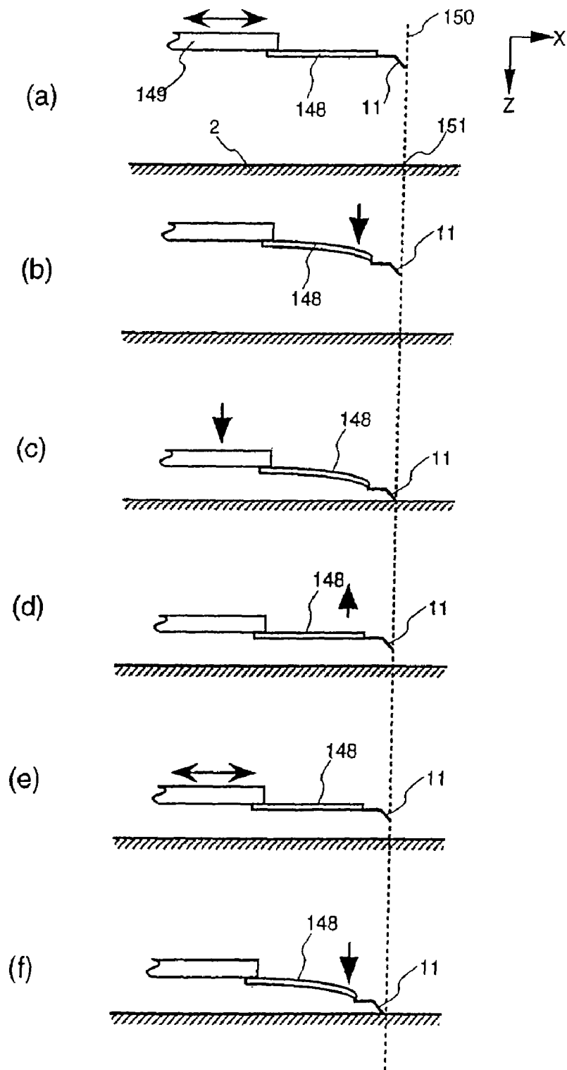
FIG.29
