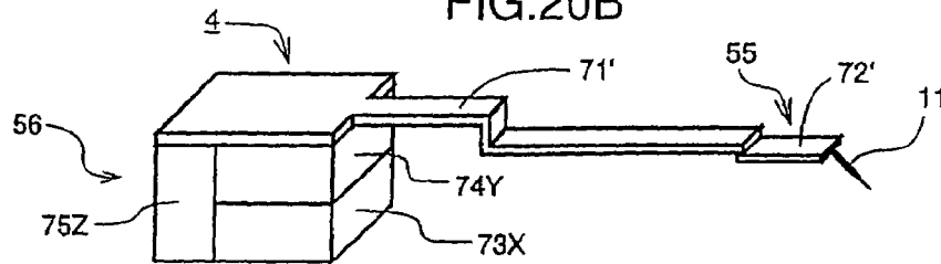
FIG.20B
