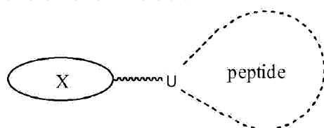
Formula 3-I-A
