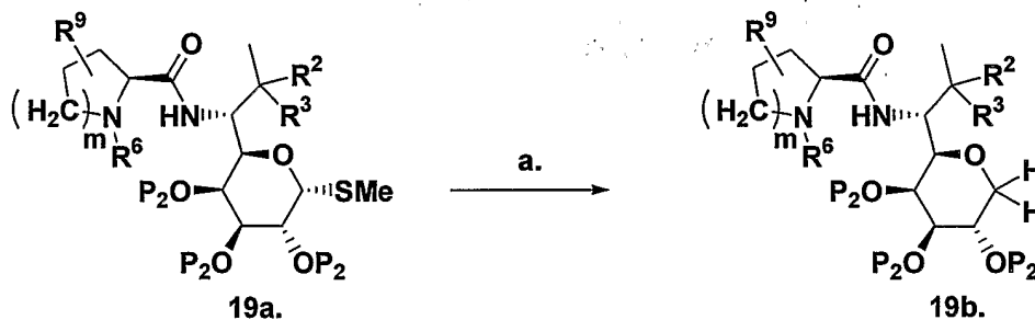
Scheme 20. a. Rainey Ni, EtOH, reflux.
