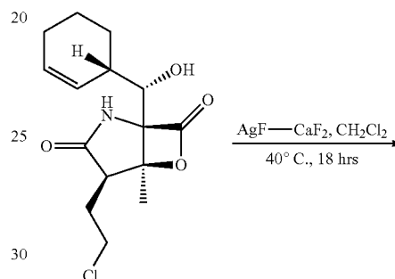
Salinosporamide A
