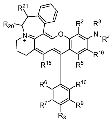
(V)
