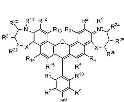
(IIa)
