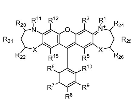
(Ia)
