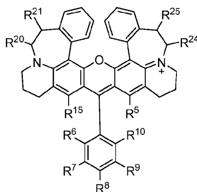
(VII)
