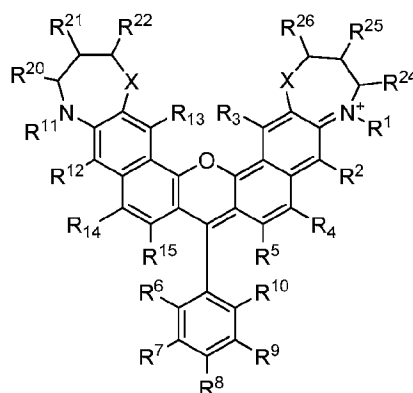
(IIb)
