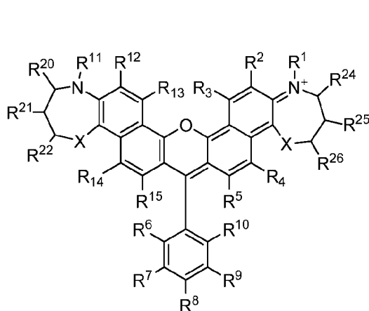
(IIa)
