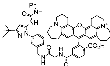
PBI-4838
