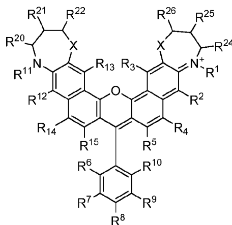
(IIb)
