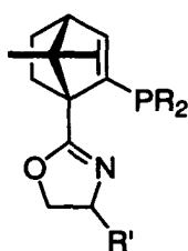
(Gilbertson)
