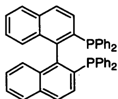
BINAP (Noyori)
