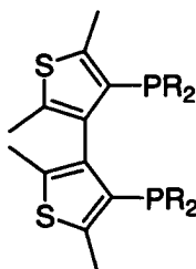
TMBTP (Sannicola)
