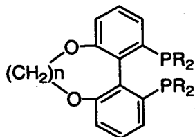
Tunaphos (Zhang)
