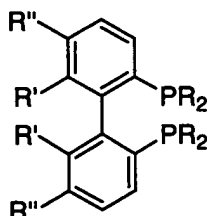
BIPHEP
