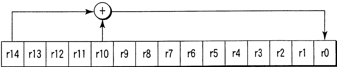
Feedback shift register
