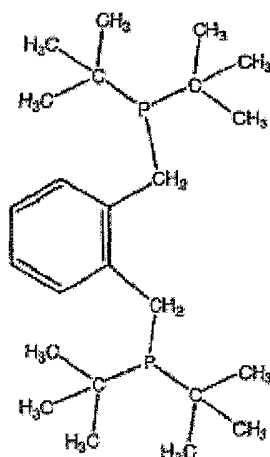
1,2-bis(ditercbutilfosfinometil) benzeno
