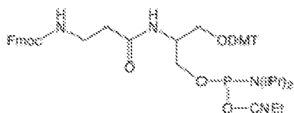
Amino-Modifier Serinol
