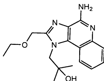
R-848
