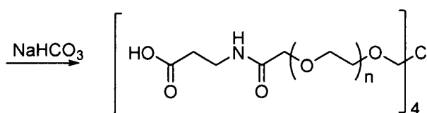
4-arm-PEG20kD-CM-beta-alanine
