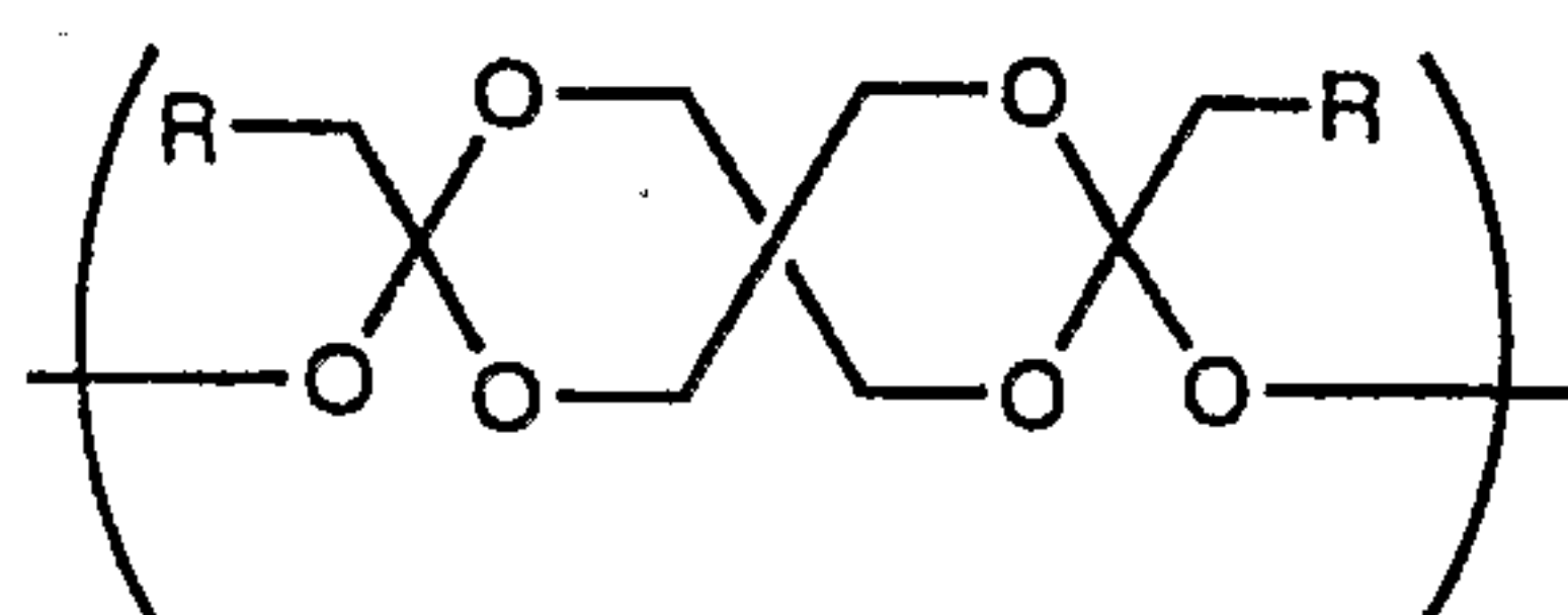
Poly(ortho ester)
