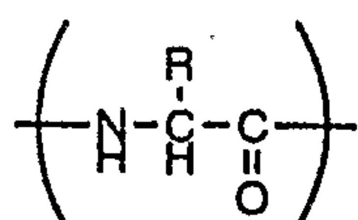
Poly(amino acid)
