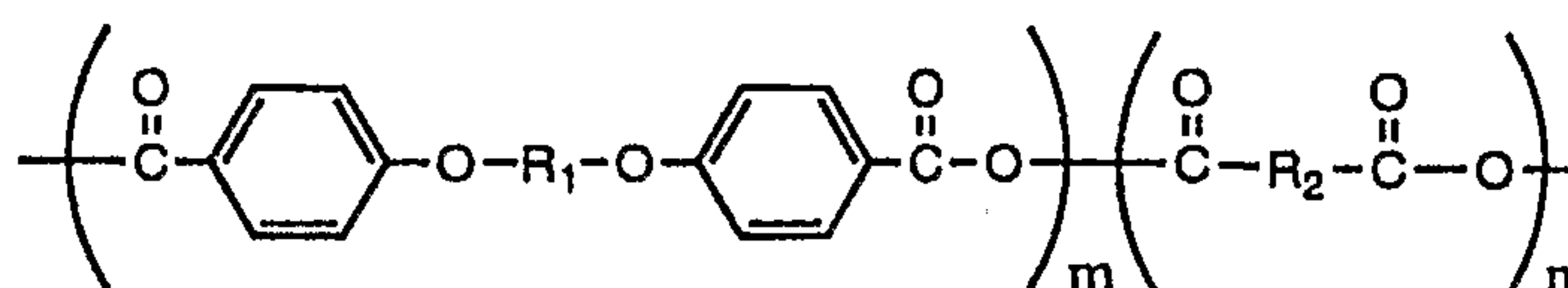
Polyanhydride
