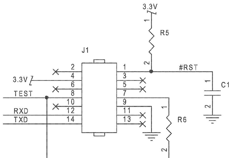
FIG. 3F
