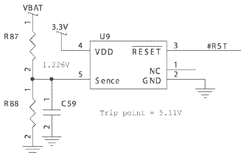
FIG. 2F
