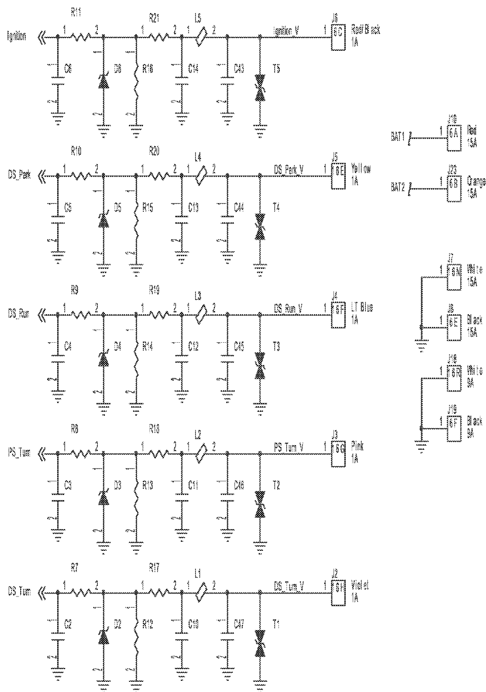
FIG. 3J
