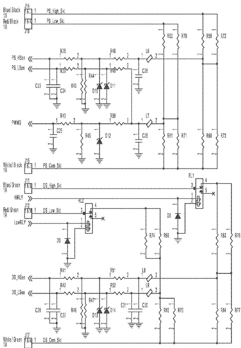
FIG. 3H
