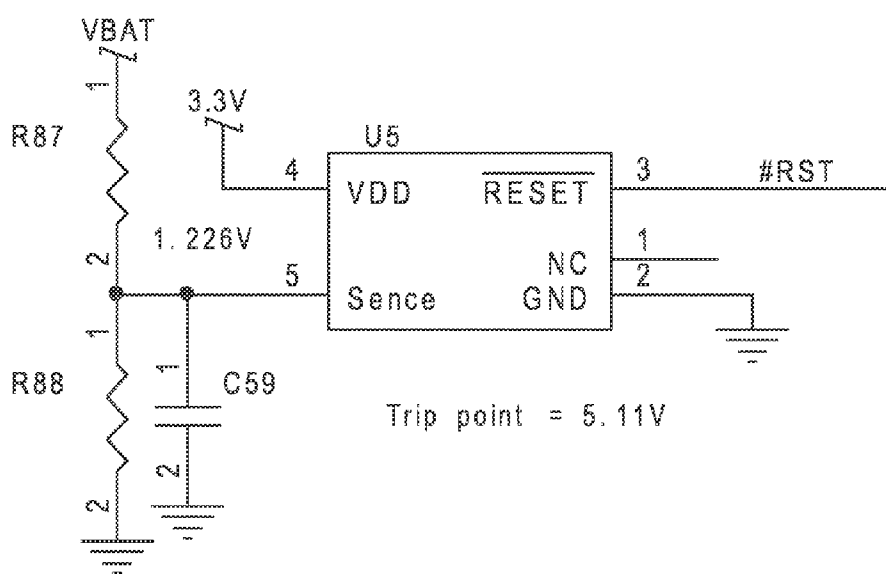
FIG. 3G
