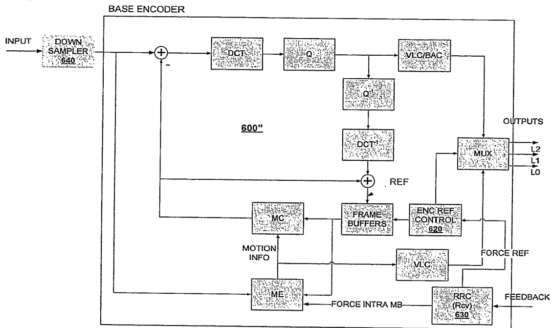
FIG. 8: SPATIAL SCALABILITY ENHANCEMENT LAYER CODEC
