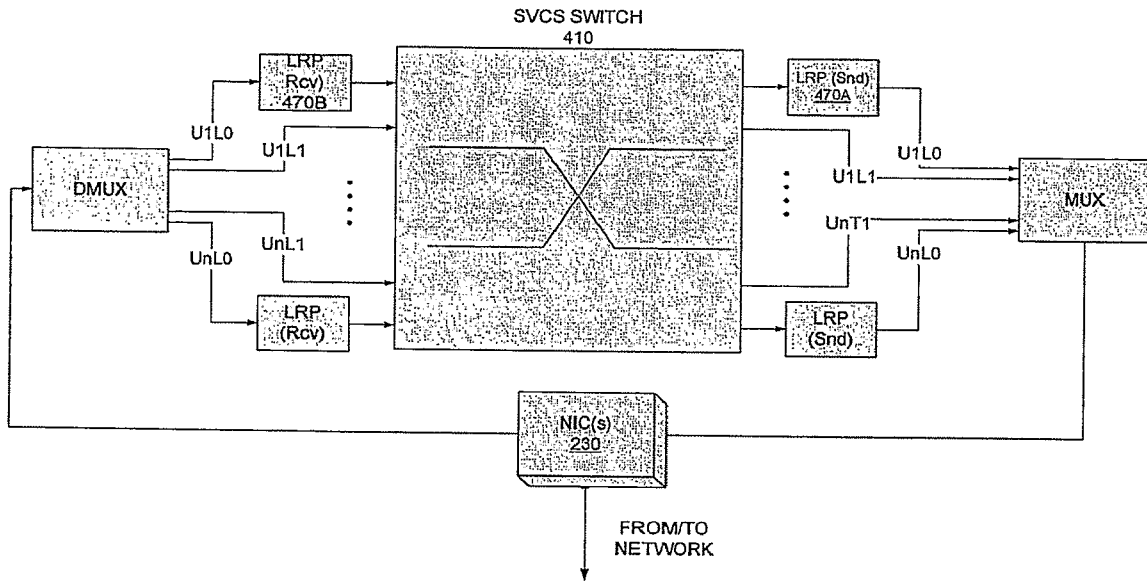
FIG. 4: SVCS
