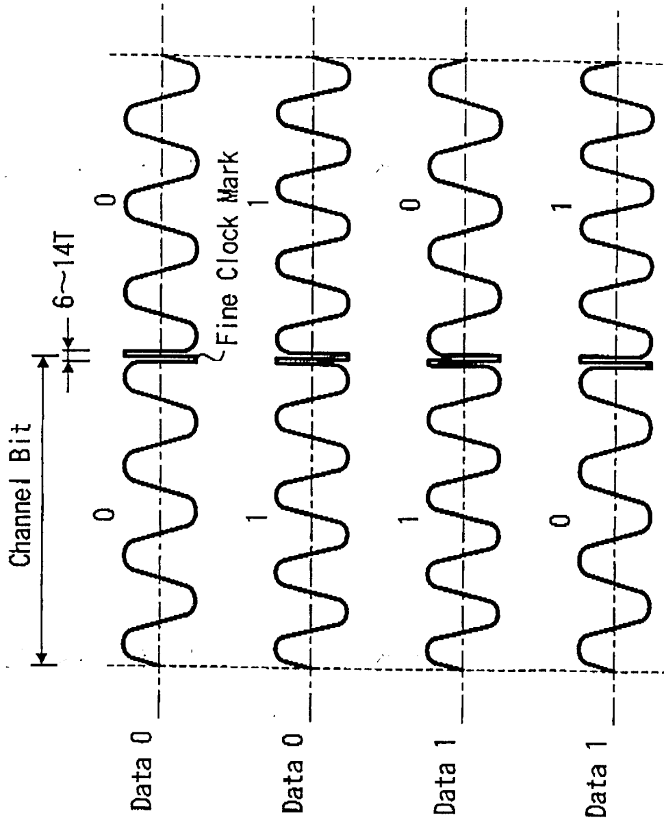
FIG. 21A
