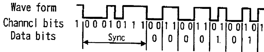
FIG. 18
