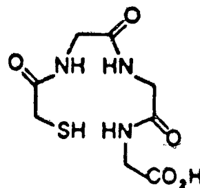
MAG 3 N 3 S triamidethiol
