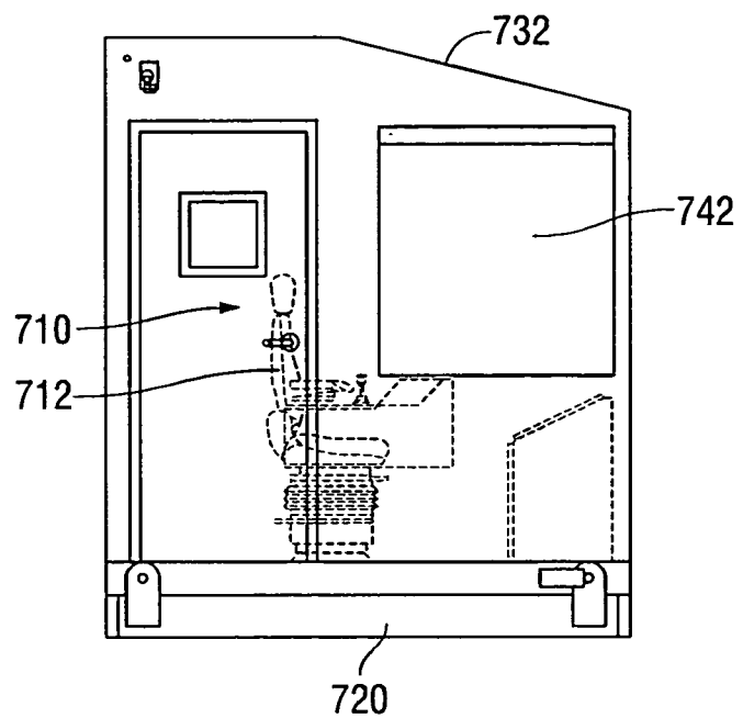
FIG. 12C
