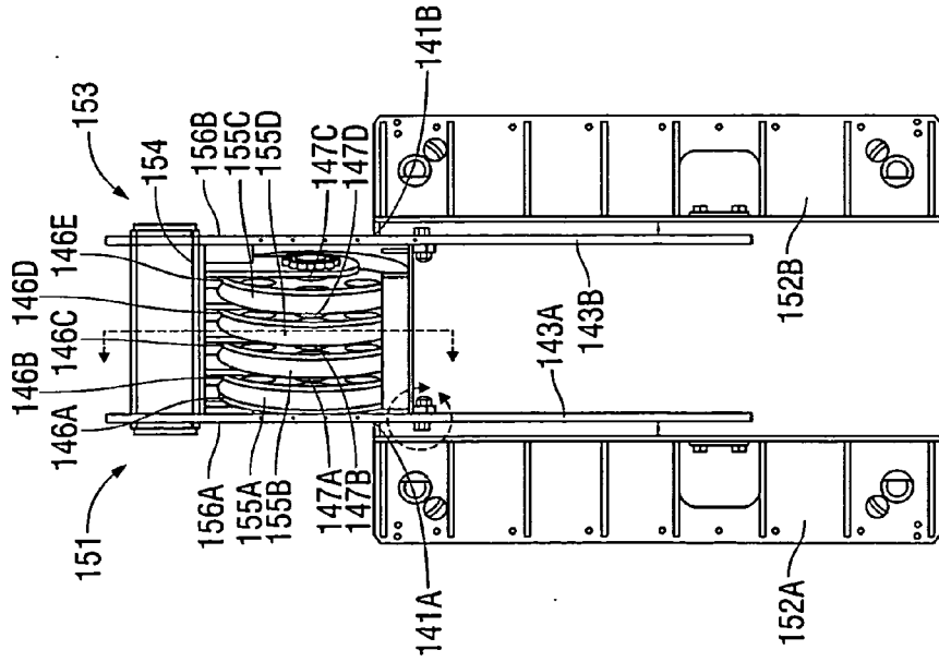
FIG. 19A
