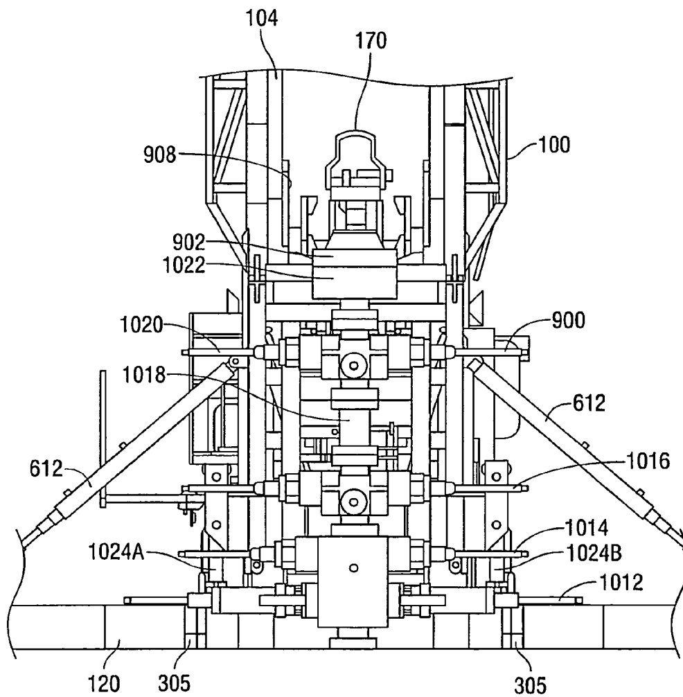
FIG. 9C-C
