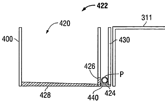
FIG. 23E
