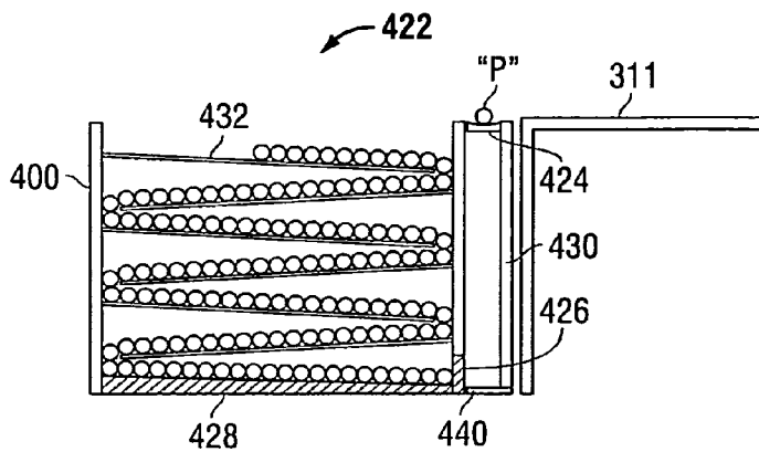
FIG. 23C
