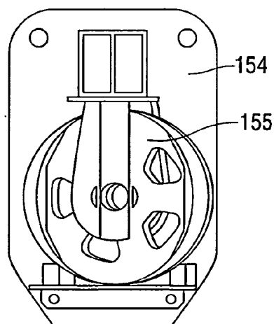
FIG. 19E-E
