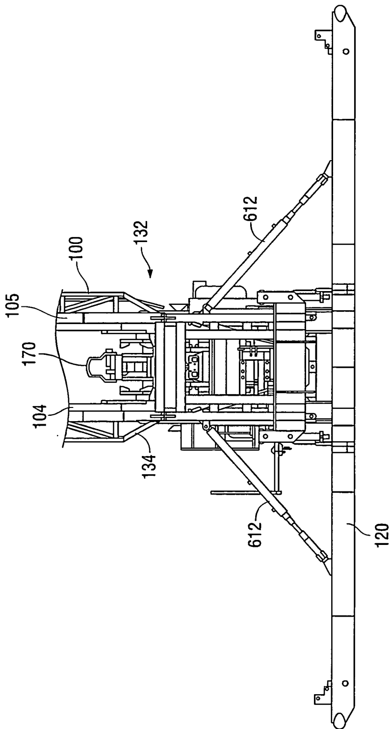
FIG. 8A-A
