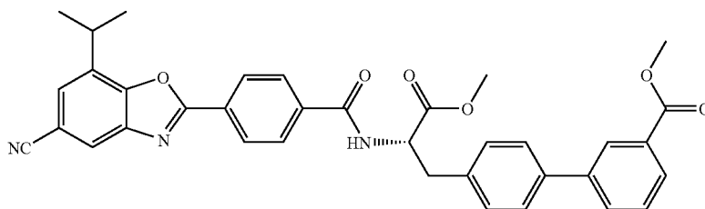
4'-((2S)-2-[[4-(5-cyano-7-isopropyl-1,3-benzoxazol-2-yl)benzoyl]amino]-3-methoxy-3-oxopropyl)biphenyl-3-carboxylate
