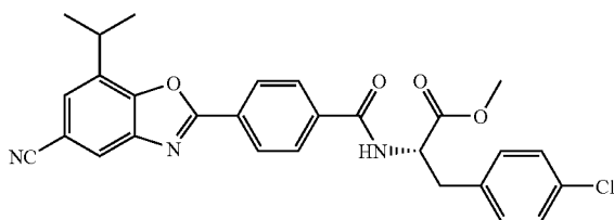
Methyl (2S)-3-(4-chlorophenyl)-2-[[4-(5-cyano-7-isopropyl-1,3-benzoxazol-2-yl)benzoyl]amino]propanoate
