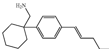
1-(1-{4-[(1E)-Pent-1-en-1-yl]phenyl}cyclohexyl)methanamine
