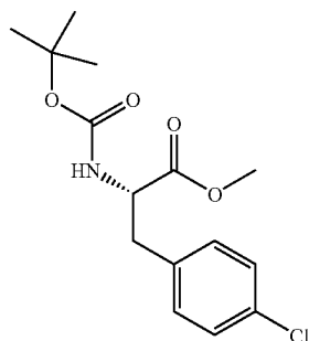
Methyl (2S)-2-[(tert-butoxycarbonyl)amino]-3-(4-chlorophenyl)propanoate
