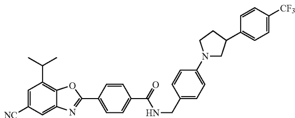
4-(5-cyano-7-isopropyl-1,3-benzoxazol-2-yl)-N-(4-{3-[4-(trifluoromethyl)phenyl]pyrrolidin-1-yl}benzyl)benzamide
