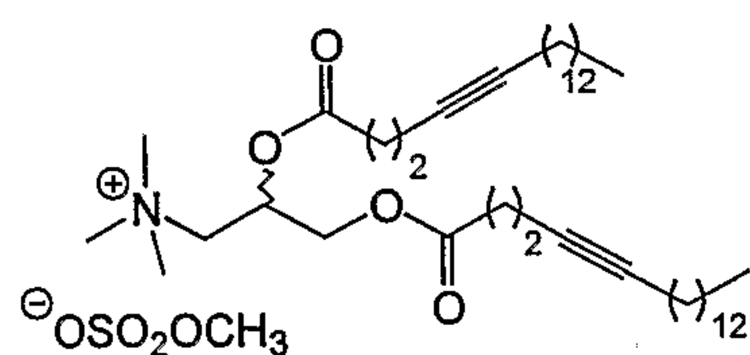
DO(4-yne)TAP (47)
