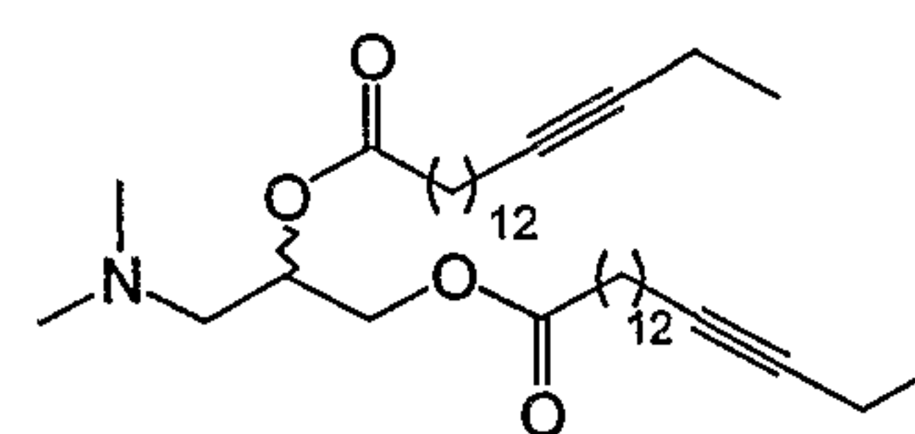
DH(14-yne)DAP (46)
