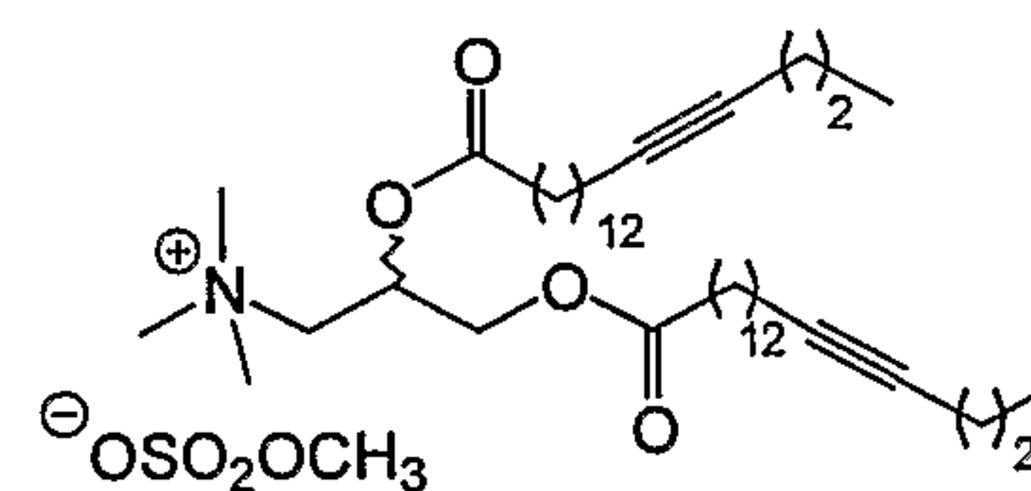
DO(14-yne)TAP (49)
