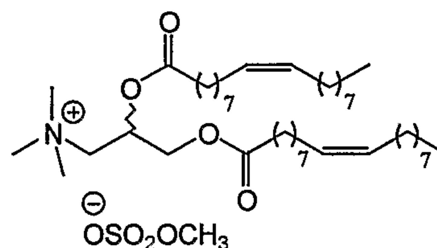
DOTAP (4)
