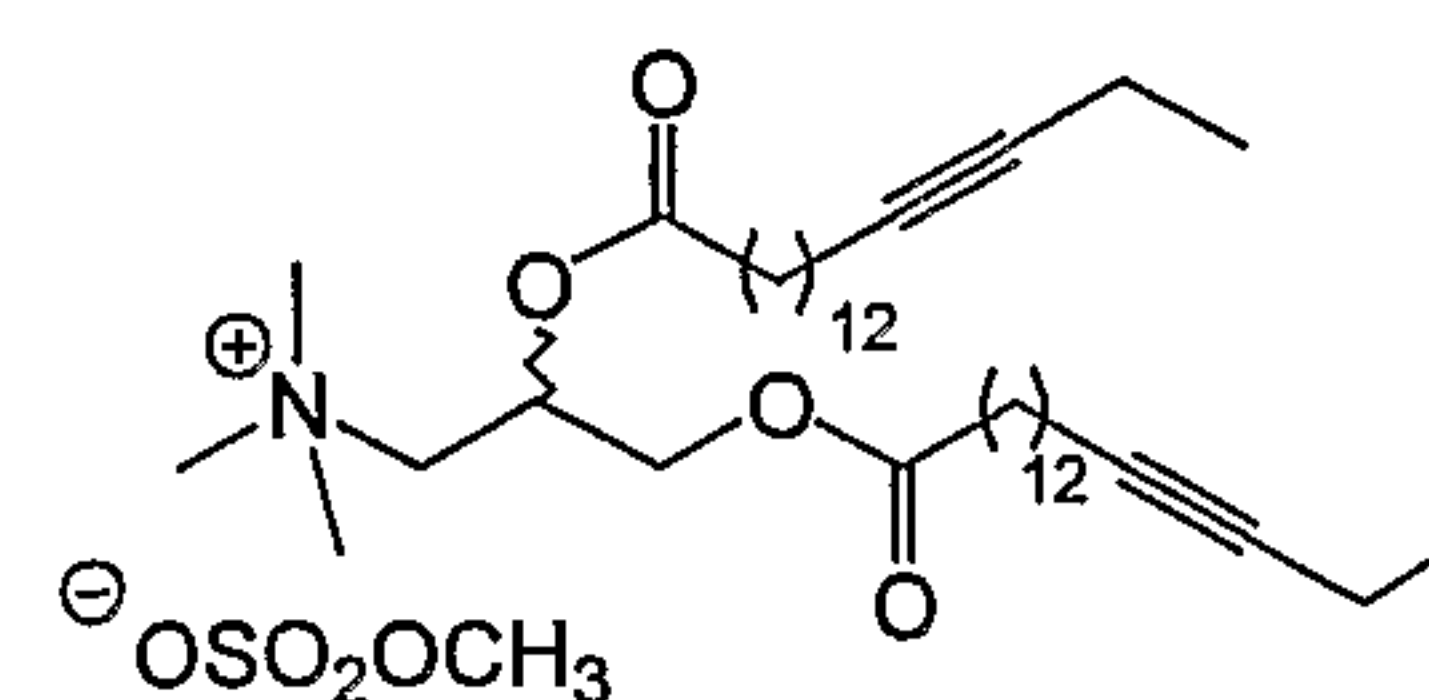
DH(14-yne)TAP (51)
