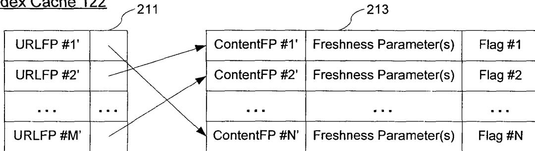
Index Cache 122
