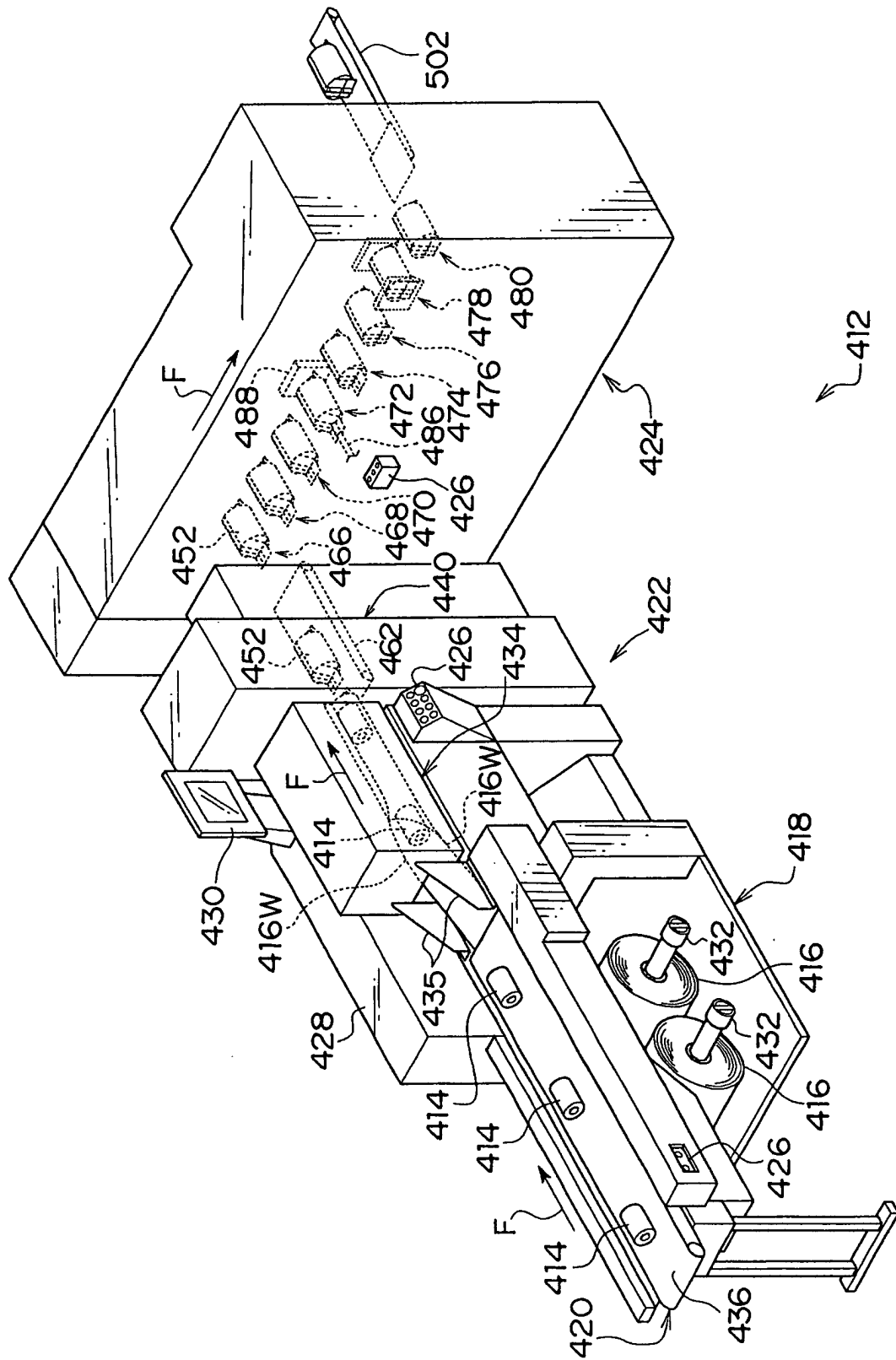
FIG. 50
