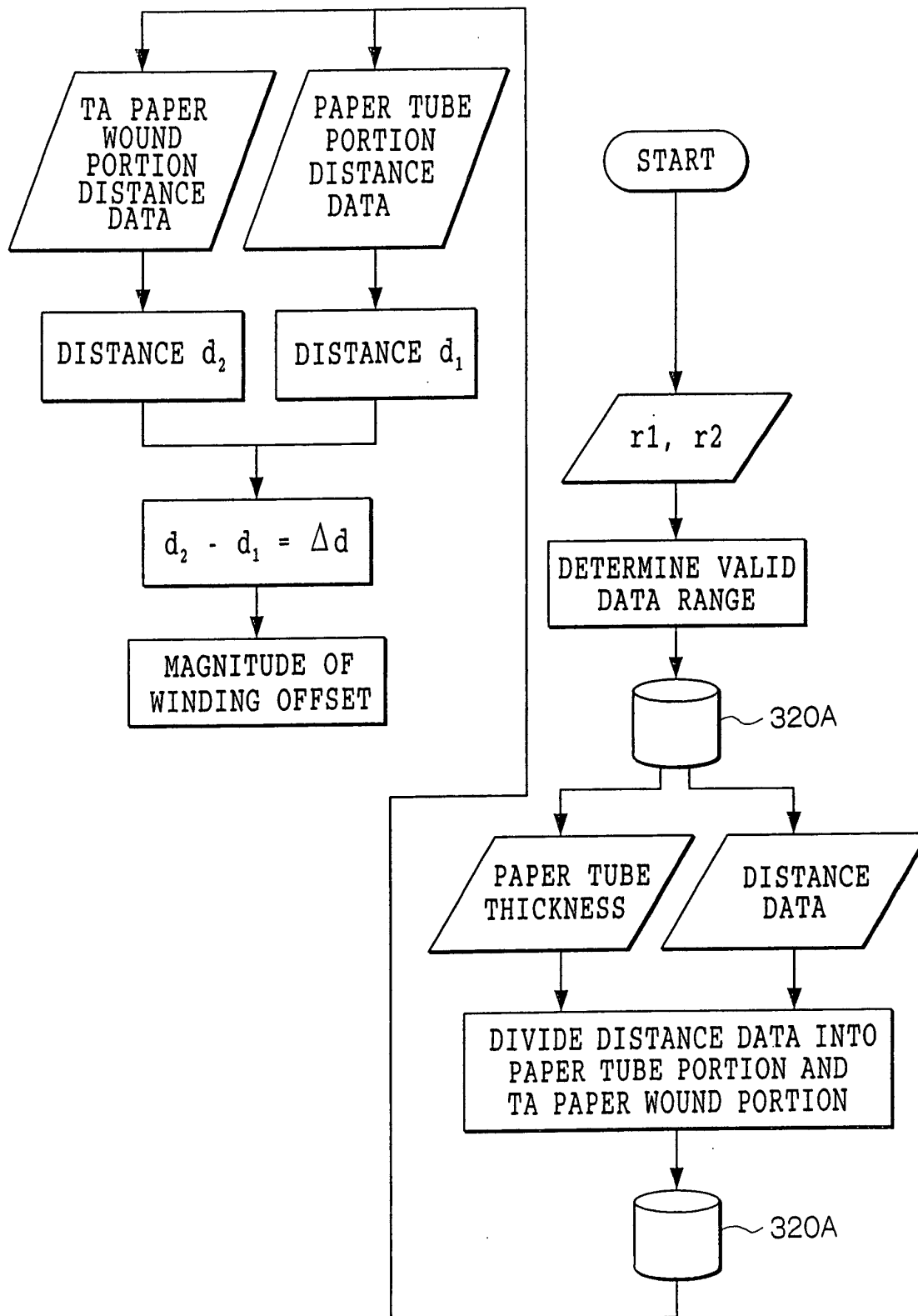
FIG.47
