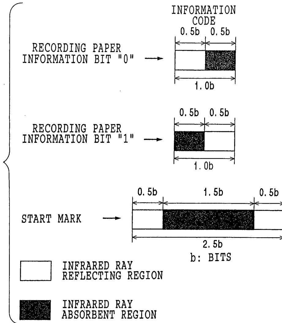
FIG.21A
