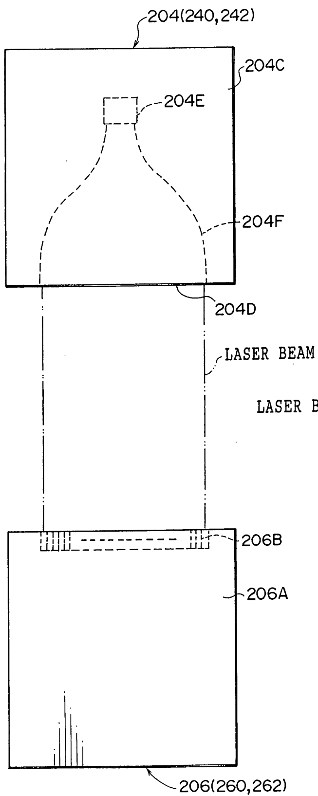
FIG.30 A
