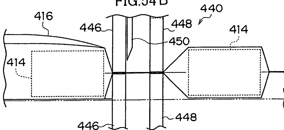
FIG.54 C
