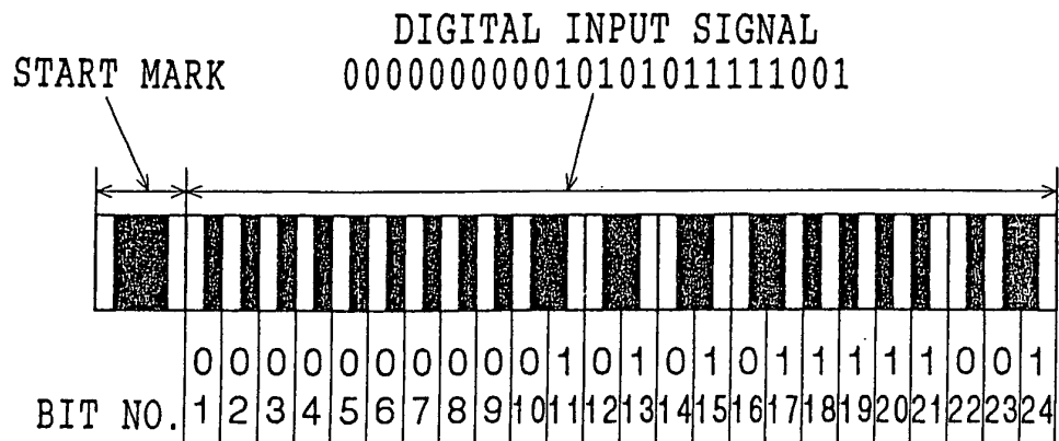
FIG.21B
