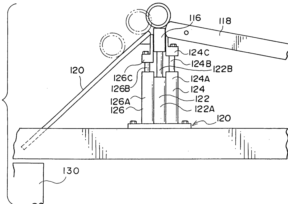
FIG.19B
