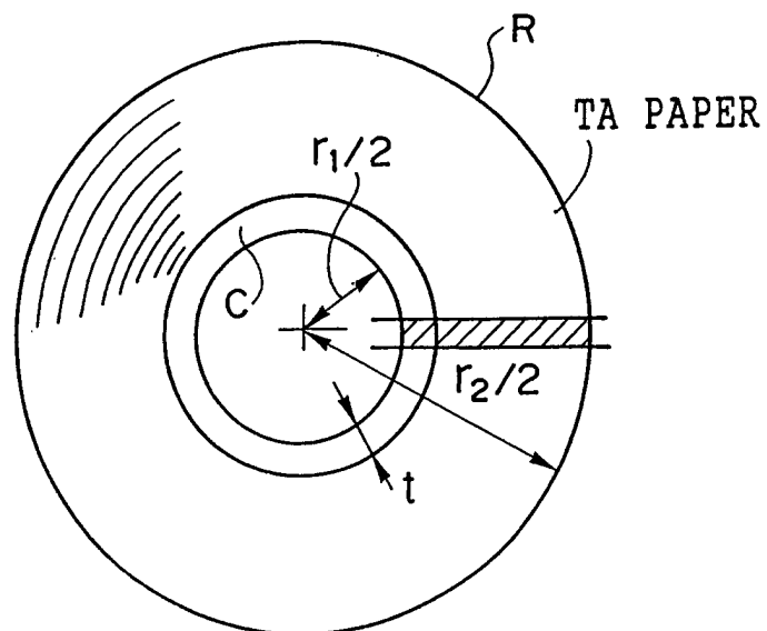
FIG.45B
