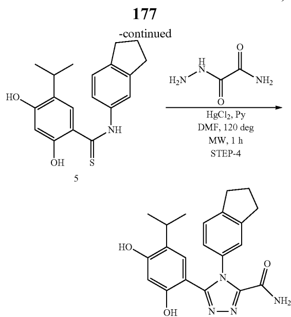
Scheme VI
