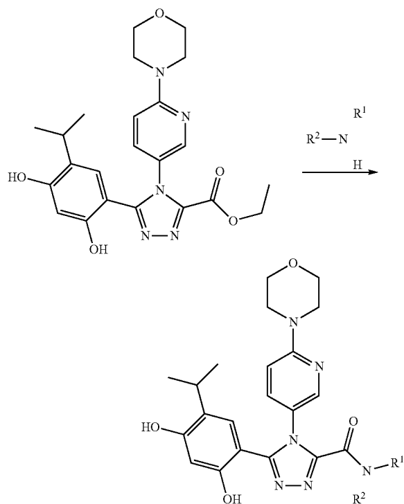
Scheme VI
