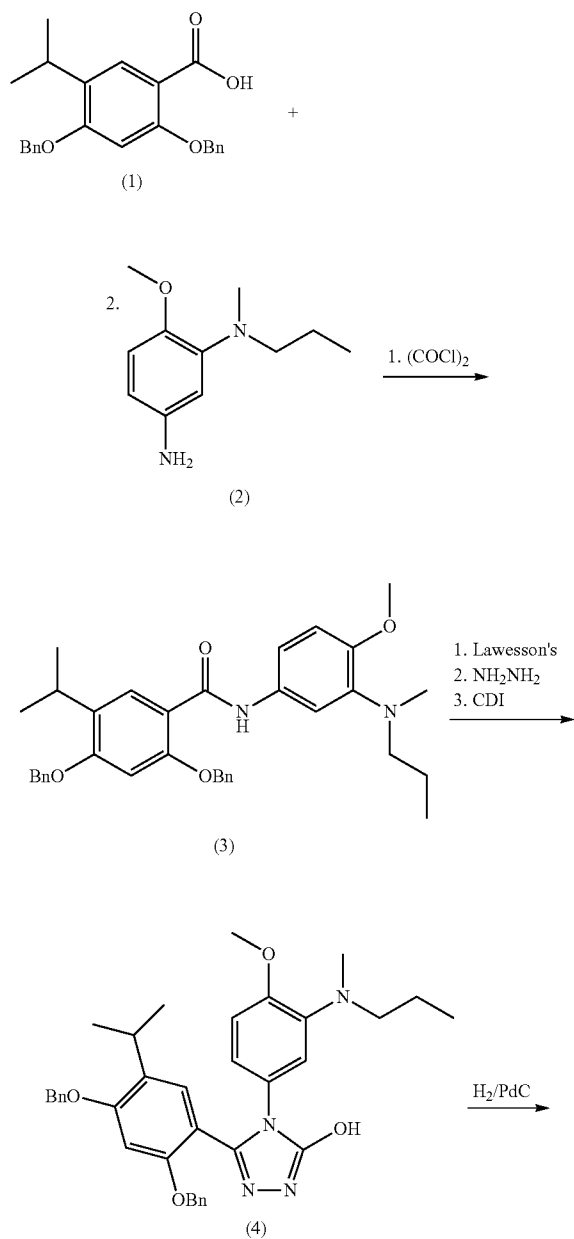
Scheme I:
