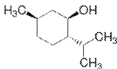
L-Menthol (MW = 156.27 Da)
