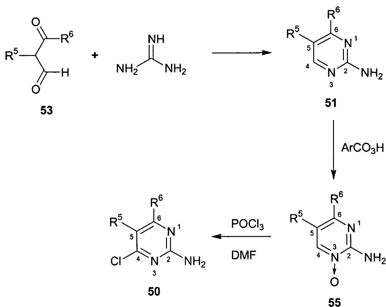
Scheme (Va)
