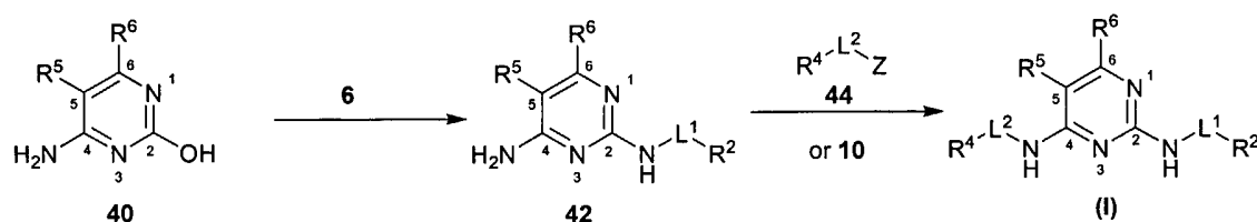
Scheme (IV)
