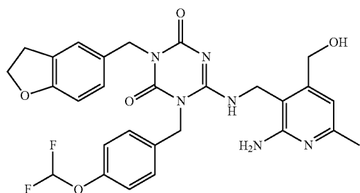
Cpd 251
