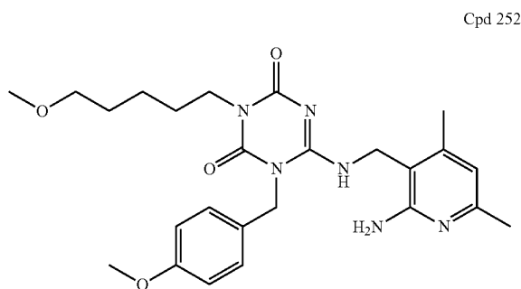
Cpd 252
