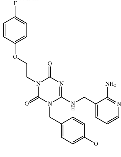
Cpd 141
