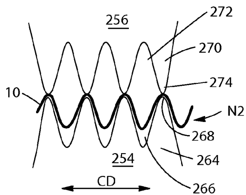
Fig. 21B
