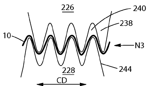
Fig. 19C
