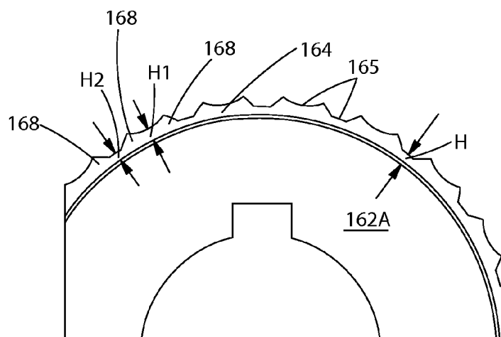
Fig. 14D
