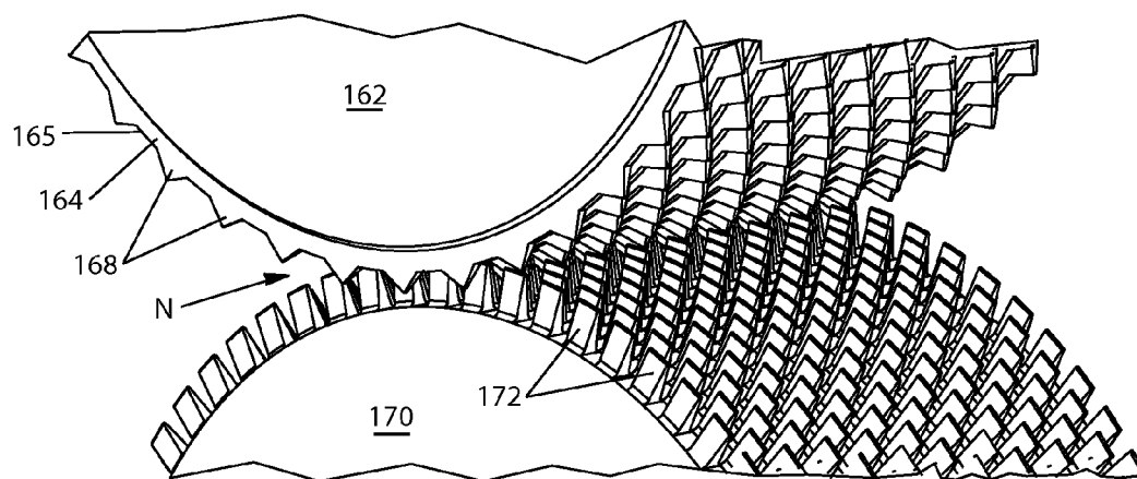
Fig. 14C
