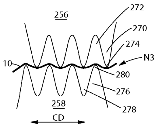
Fig. 21C
