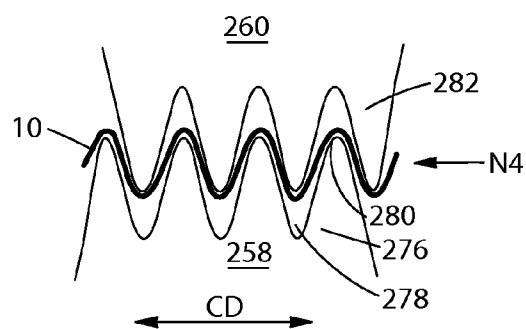
Fig. 21D
