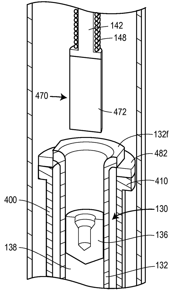
FIG. 8B
