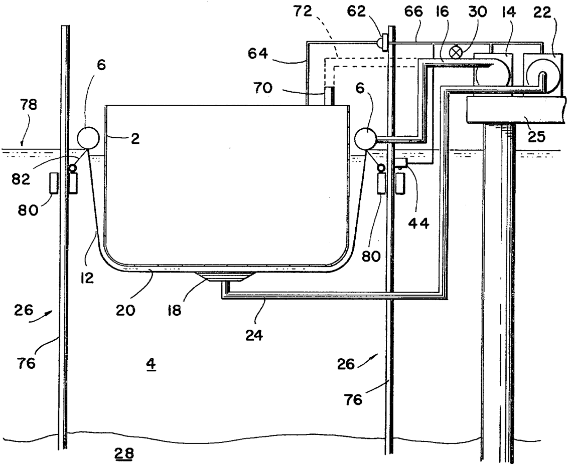
FIG. 2 SEC. A - A'
