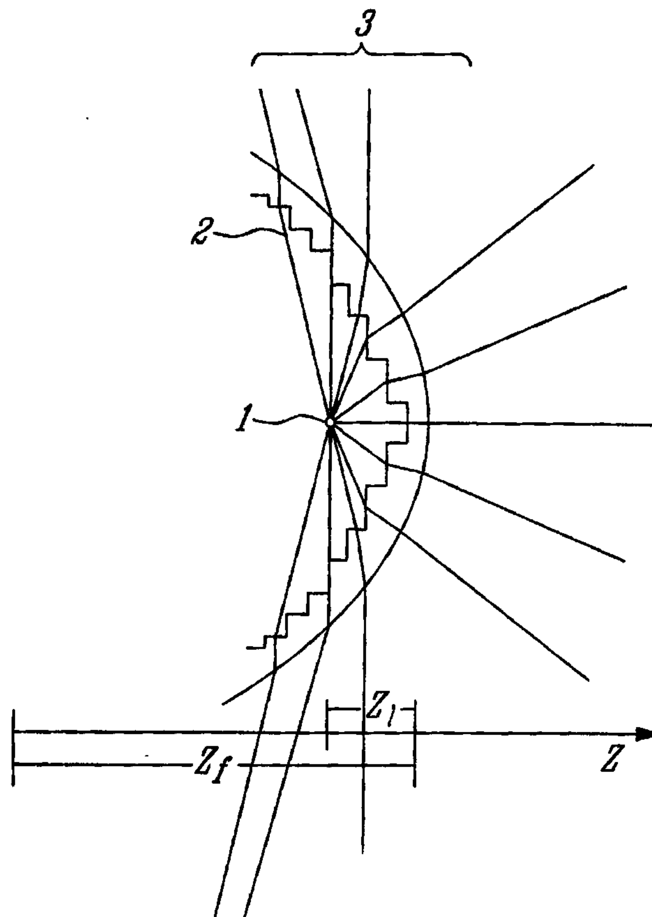
FIG. 1B
