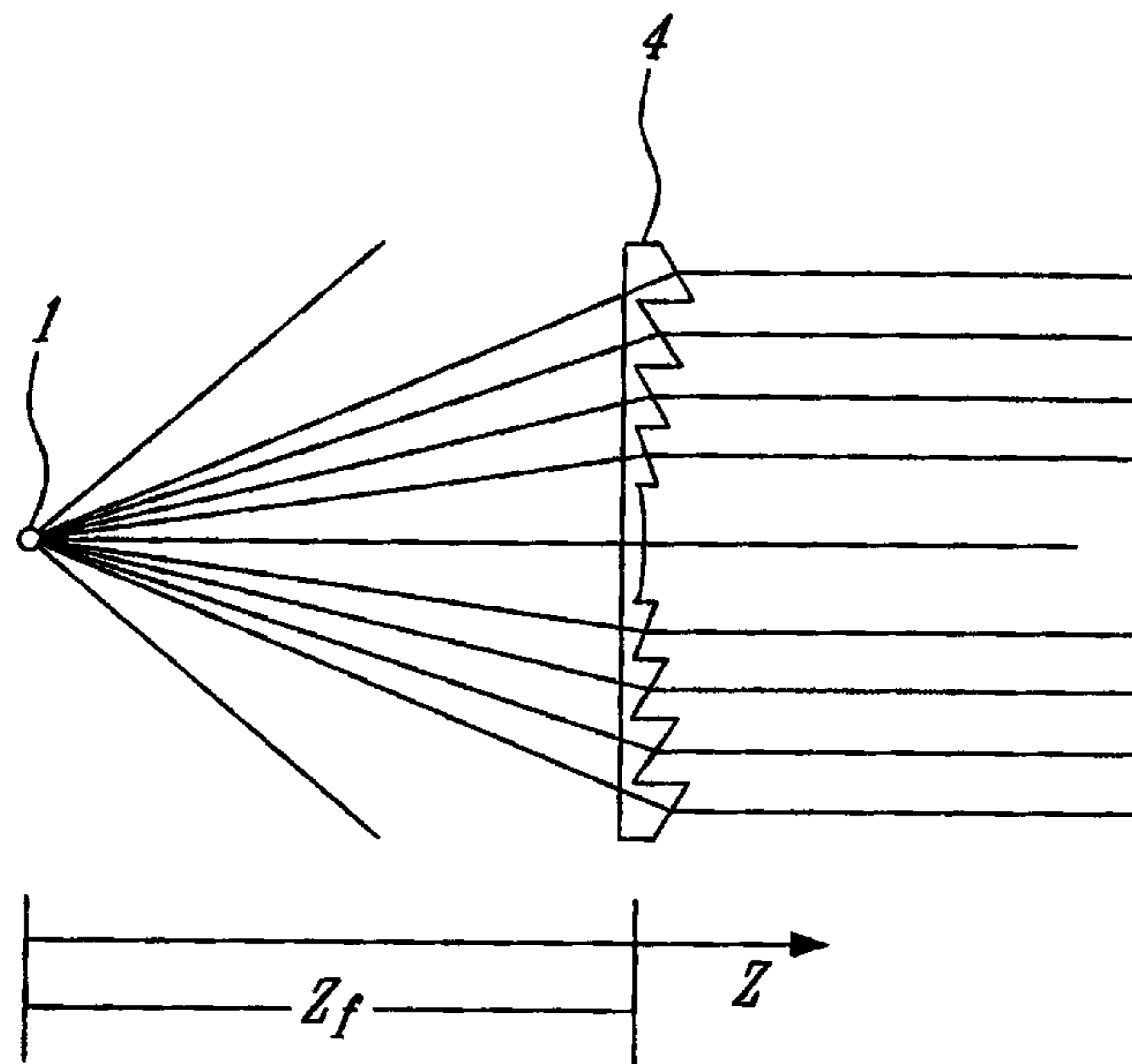
FIG. 2A
