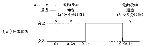
電動役物の動作態様
