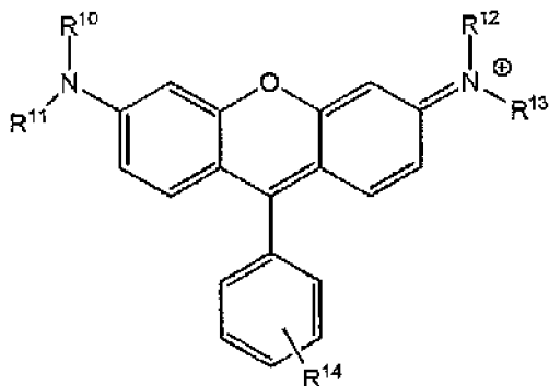
Formule générale (A4-1)
