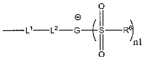
Formule générale (A4-1-1)
