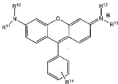
Formule générale (A4-3)
