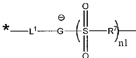
Formule générale (A3-2)
