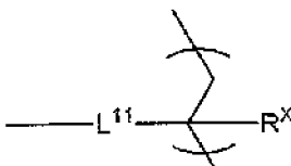
Formule générale (A4-1-2)
