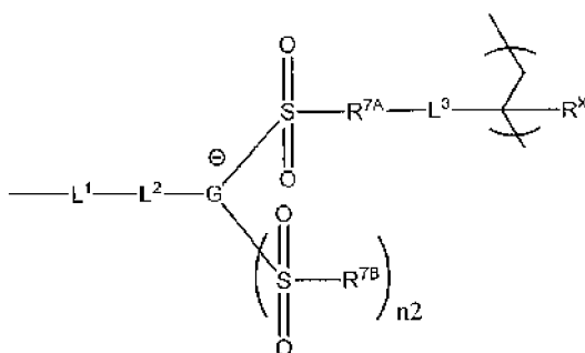
Formule générale (A4-3-1)
