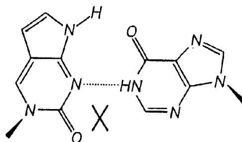
PyrroloPyr•I
