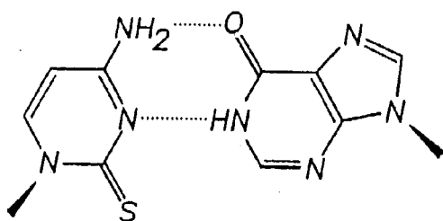
2-thioC•I
