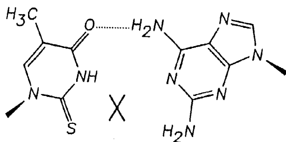
2-thioT•2-aminoA
