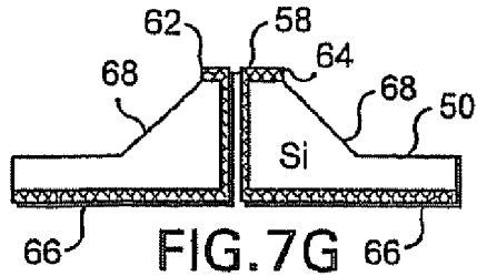
STEP 7. ANISOTROPIC ETCH
