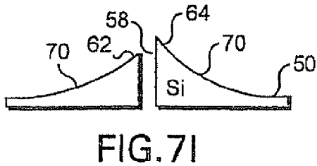
STEP 8. ISOTROPIC ETCH
