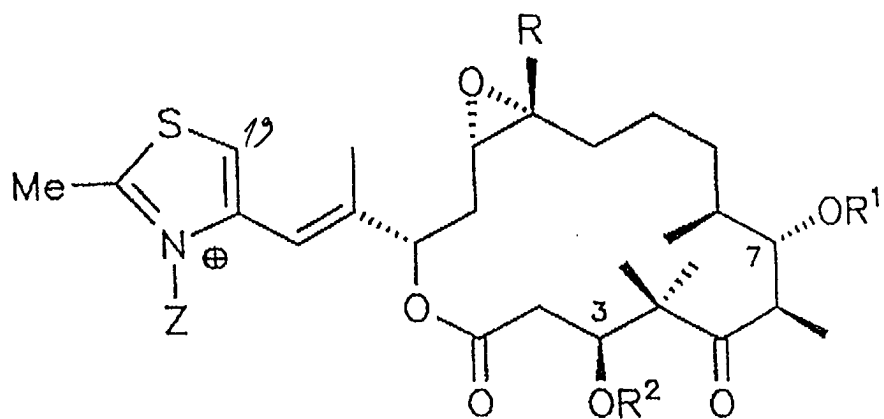
2a R^1, R^2 = H, Z = O^-, R = H
