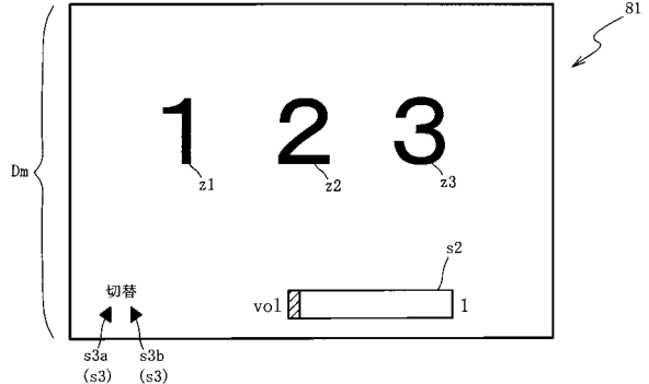
客待ち画面
