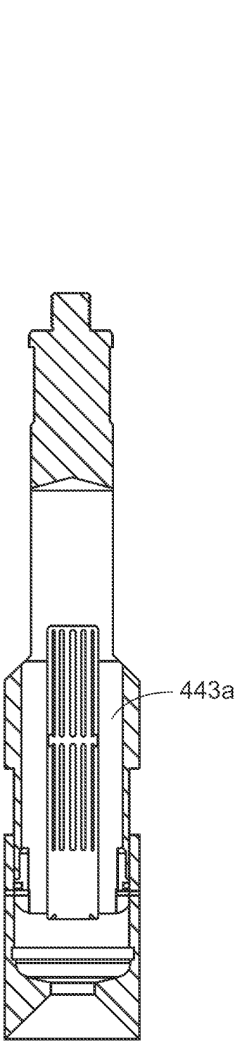
400a FIG. 4A
