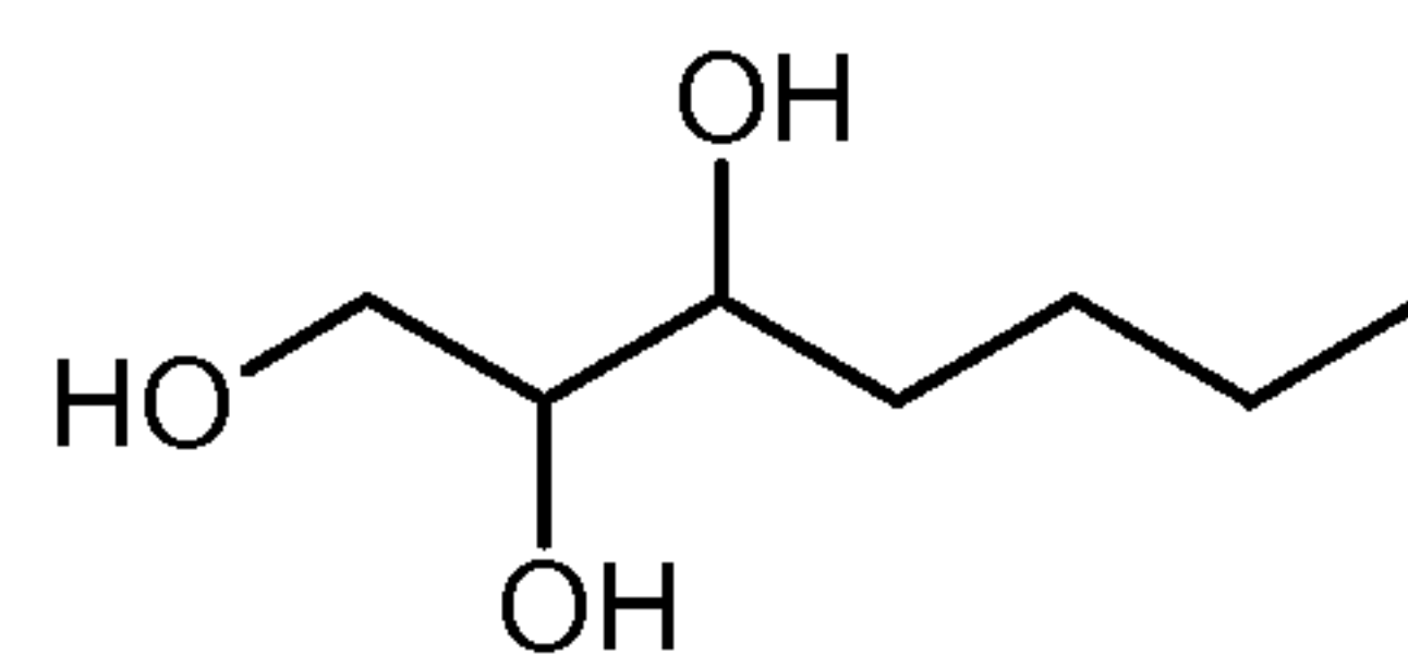
1,2,3-Heptanetriol
