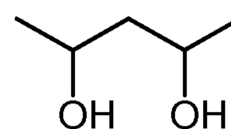
2,4-Pentanediol
