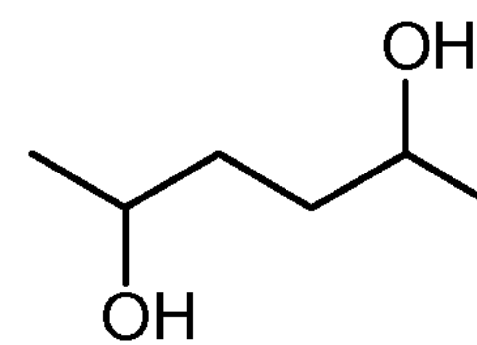
2,5-Hexanediol
