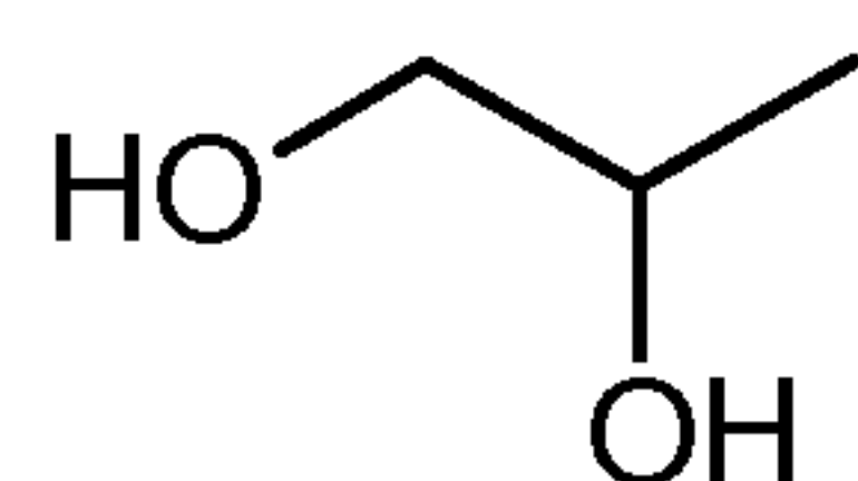
1,2-Propanediol
