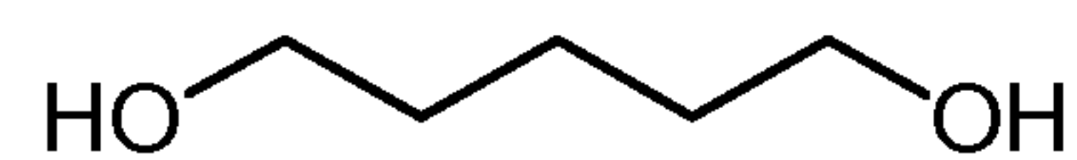
1,5-Pentanediol
