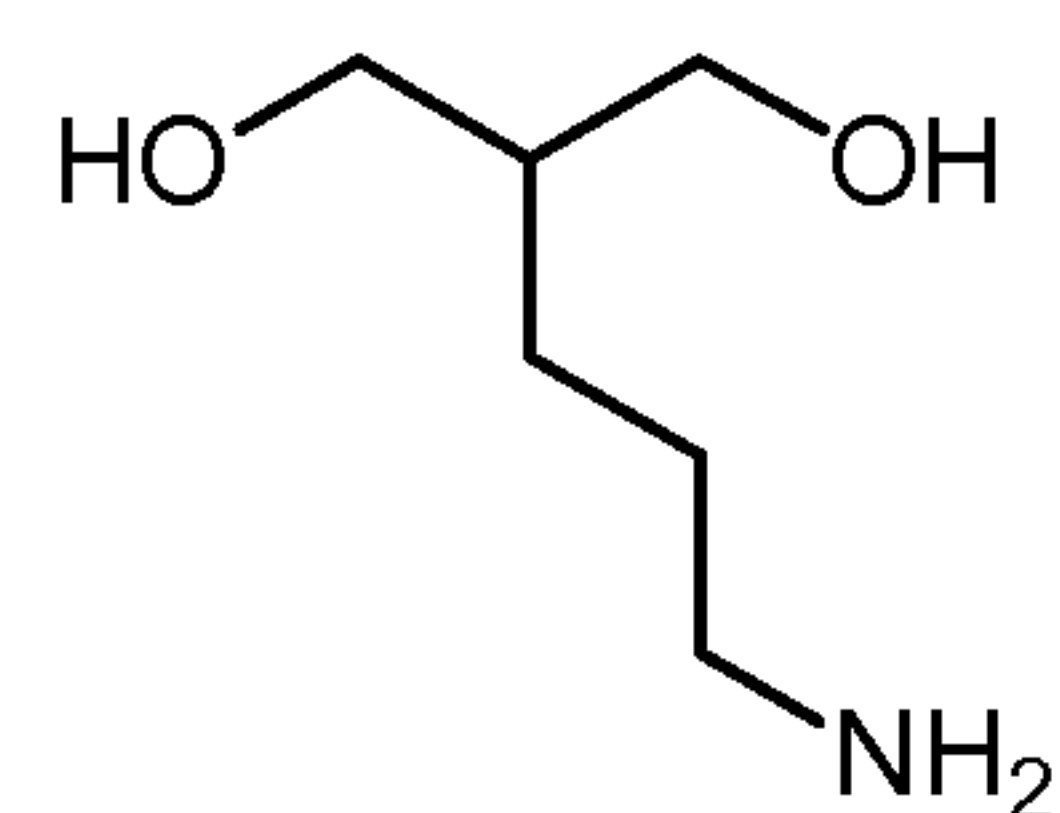
2-(1-Aminopropyl)-1,3-propanediol
