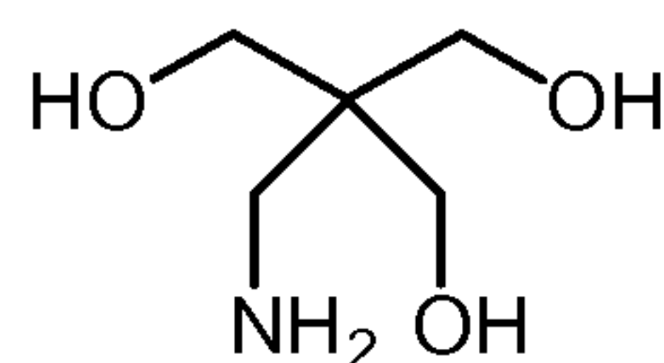
2-Amino-2-(hydroxymethyl)-1,3-propanediol
