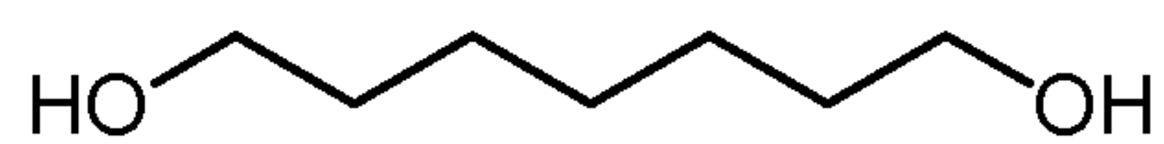
1,7-Heptanediol
