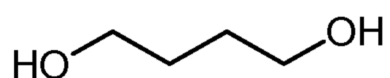
1,4-Butanediol
