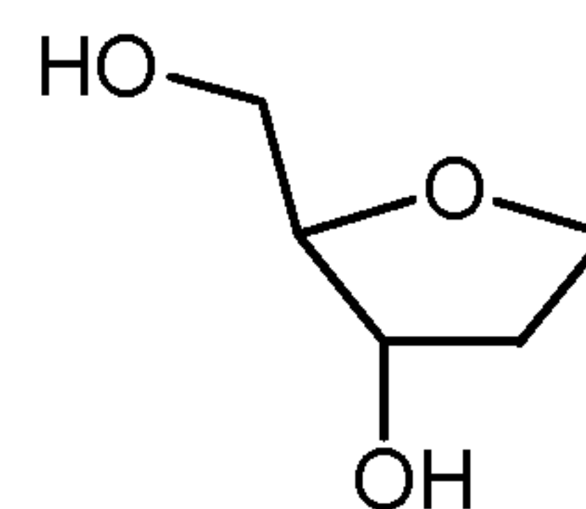
1,2-Dideoxyribose
