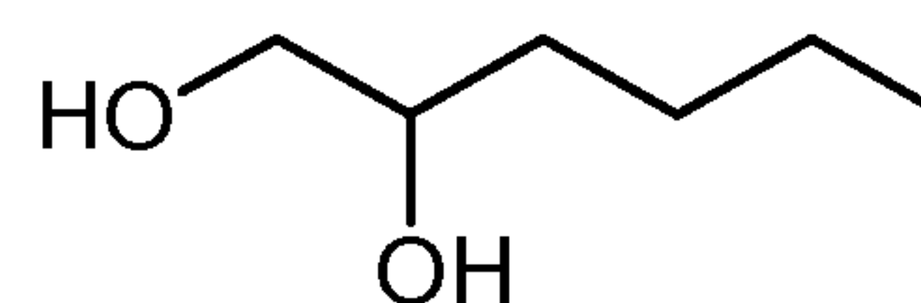
1,2-Hexanediol
