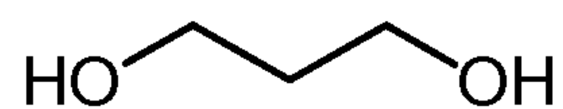
1,3-Propanediol
