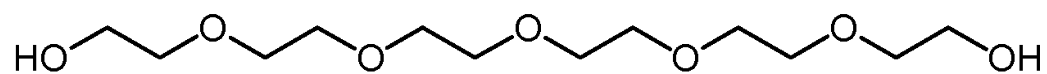
Hexaethylene glycol
