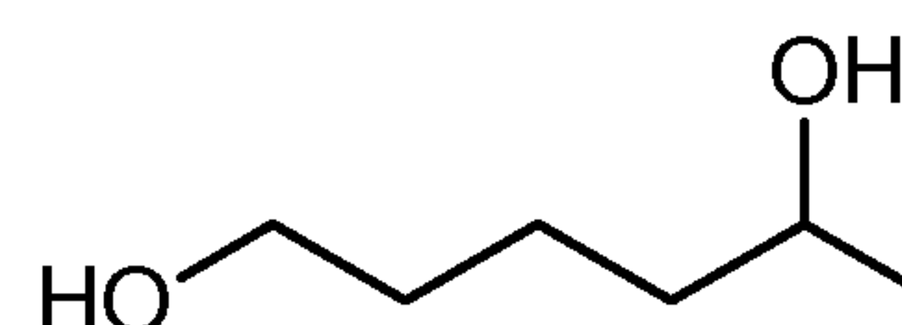
1,5-Hexanediol
