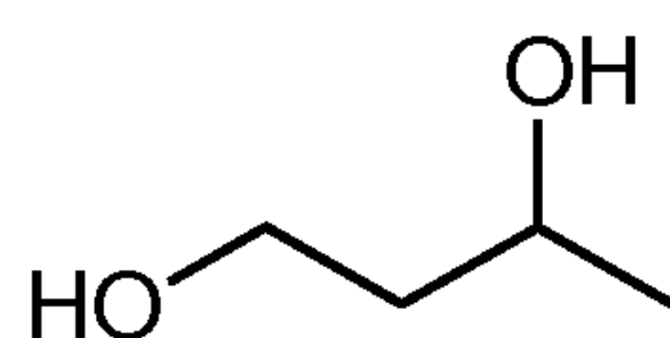
1,3-Butanediol
