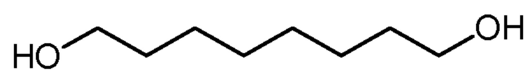
1,8-Octanediol
