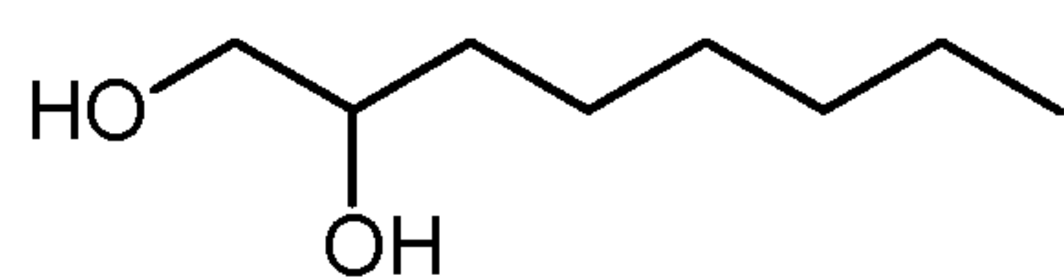
1,2-Octanediol
