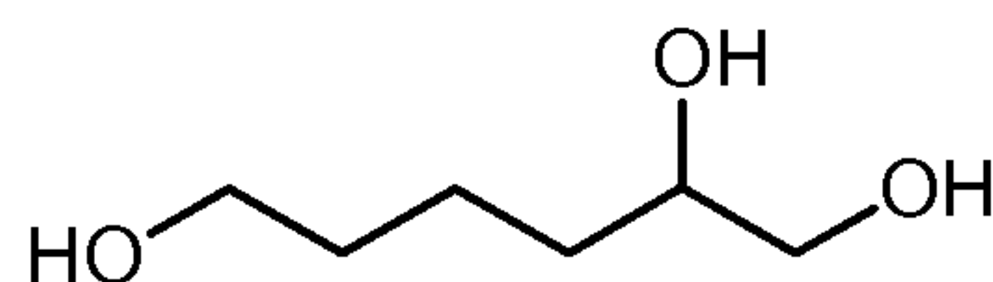
1,2,6-Hexanetriol
