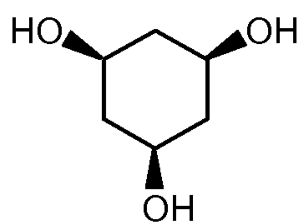
cis-1,3,5-Cyclohexanetriol
