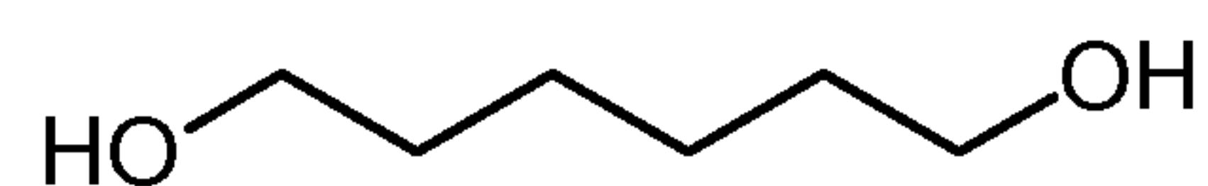
1,6-Hexanediol
