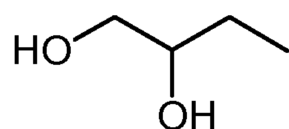
1,4-Butanediol
