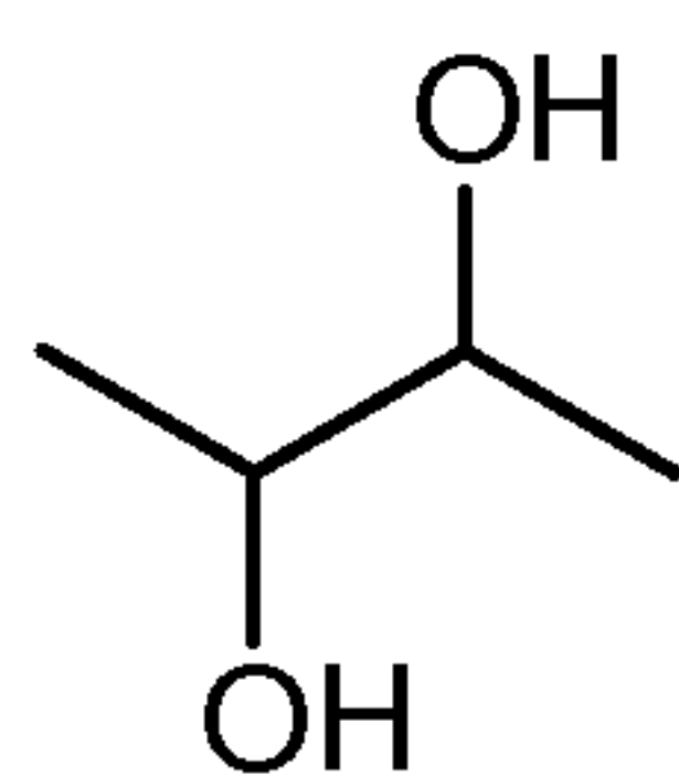
2,3-Butanediol
