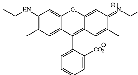
Rhodamine 575
