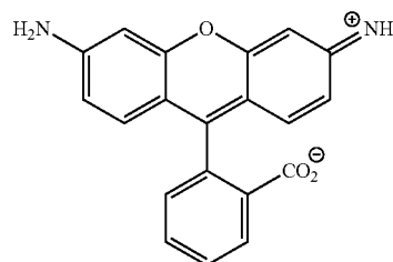
Rhodamine 110
