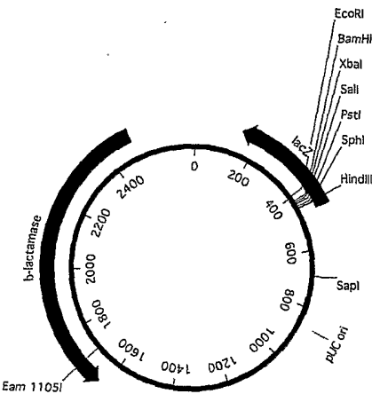
pUC 19
