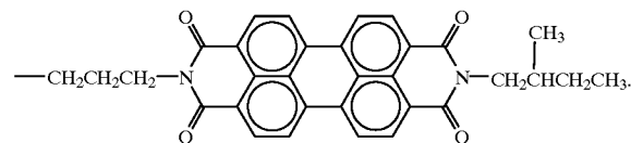
1-(n-pentylimidoperyleneimido)-3-(2-methylbutylimidoperyleneimido)propane
