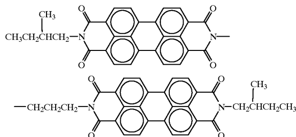
1,3-bis(2-methylbutylimidoperyleneimido)propane
