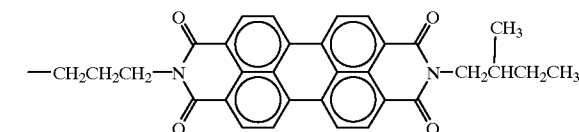
1,3-bis(2-methylbutylimidoperyleneimido)propane
