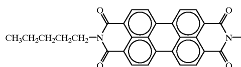
1,3-bis(2-methylbutylimidoperyleneimido)propane
