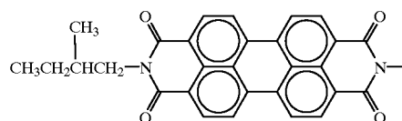
1,3-bis(n-pentylimidoperyleneimido)propane
