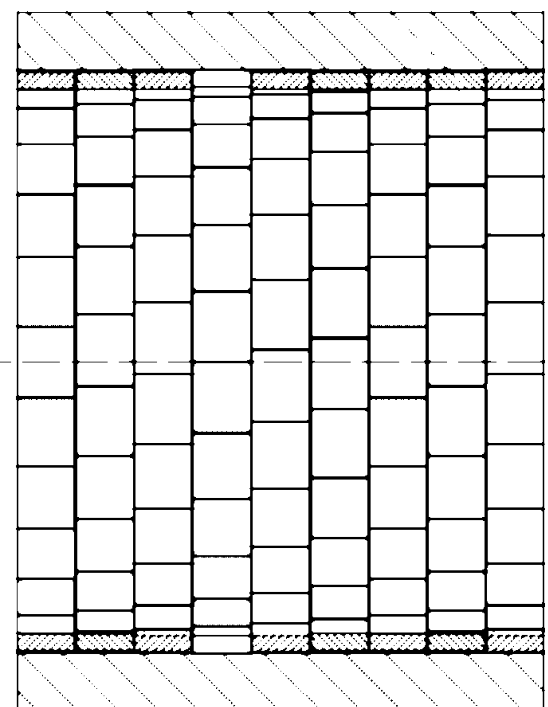
Section A-A
