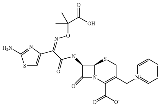
Ceftazidime
