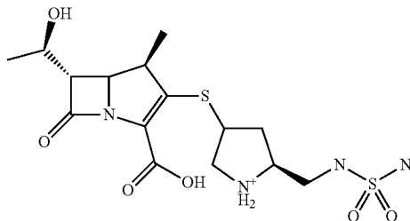
Doripenem
