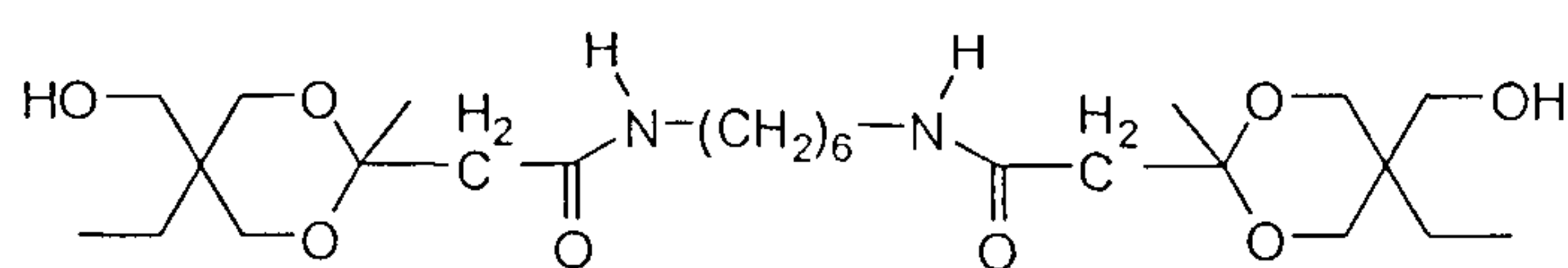
Ia
