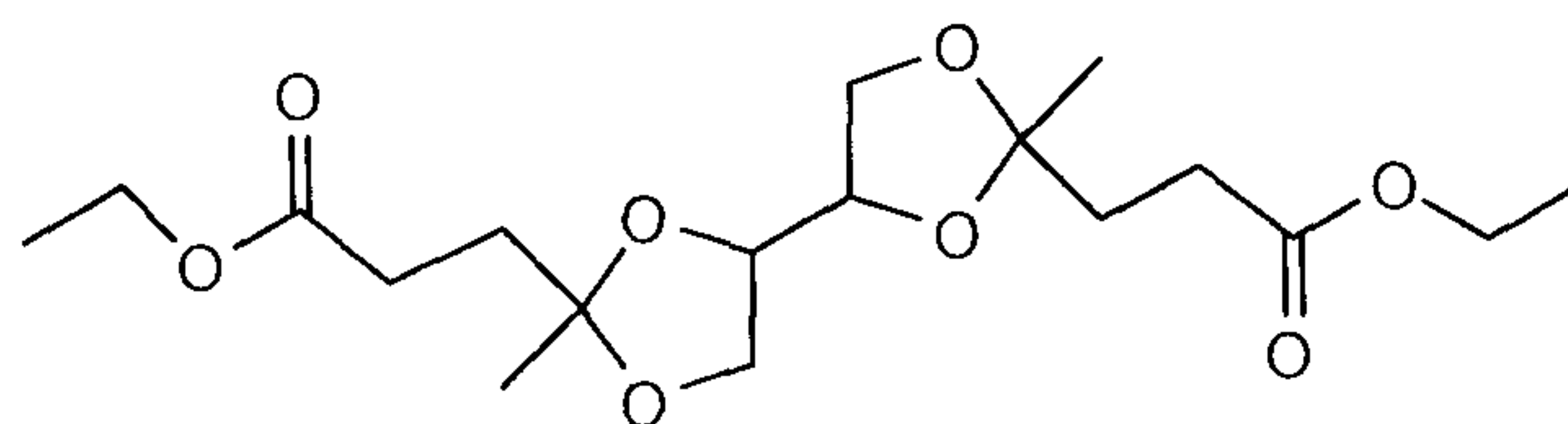
EtBLEK
