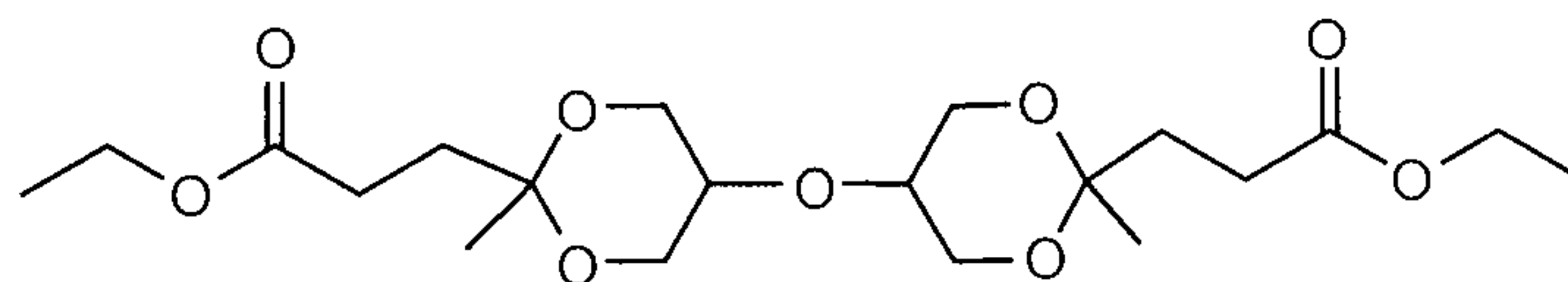
EtBLDK
