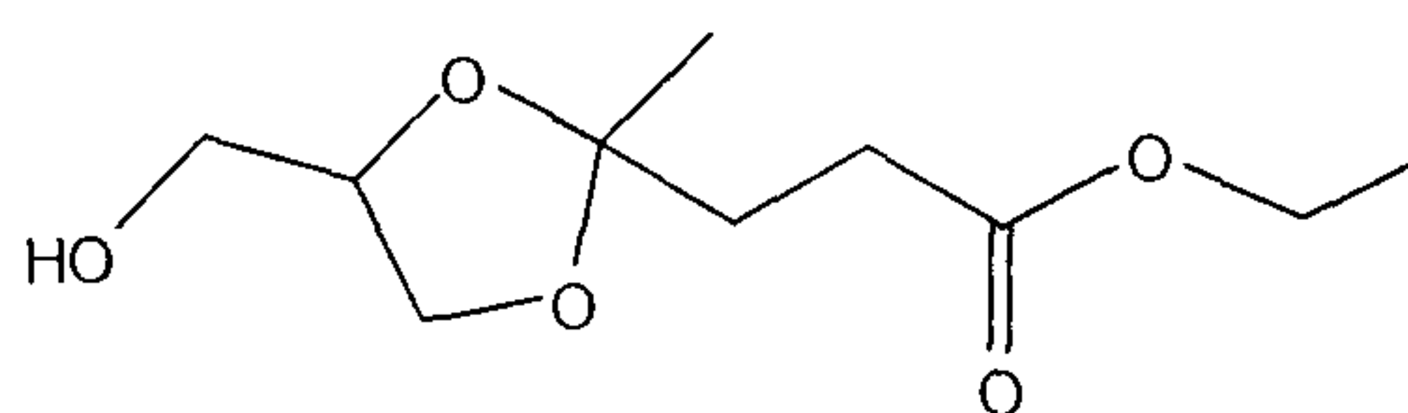
EtLGK
