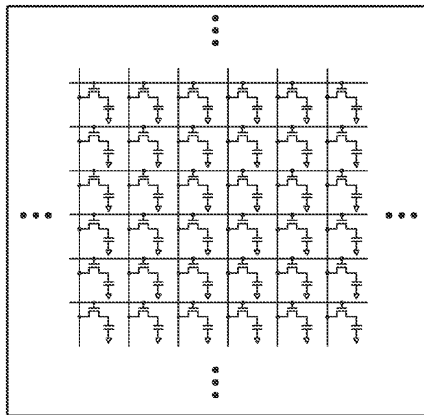
Cell Array
