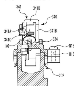
(B) T—T断面図
