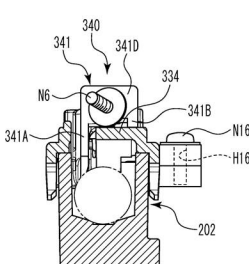
(D) U—U断面图
