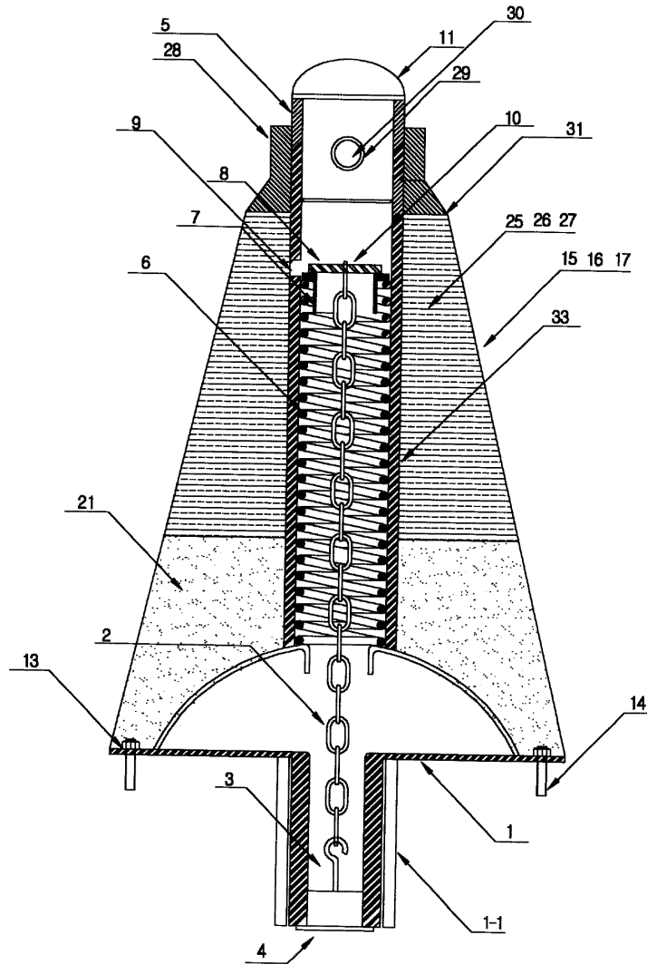
조립도-3
