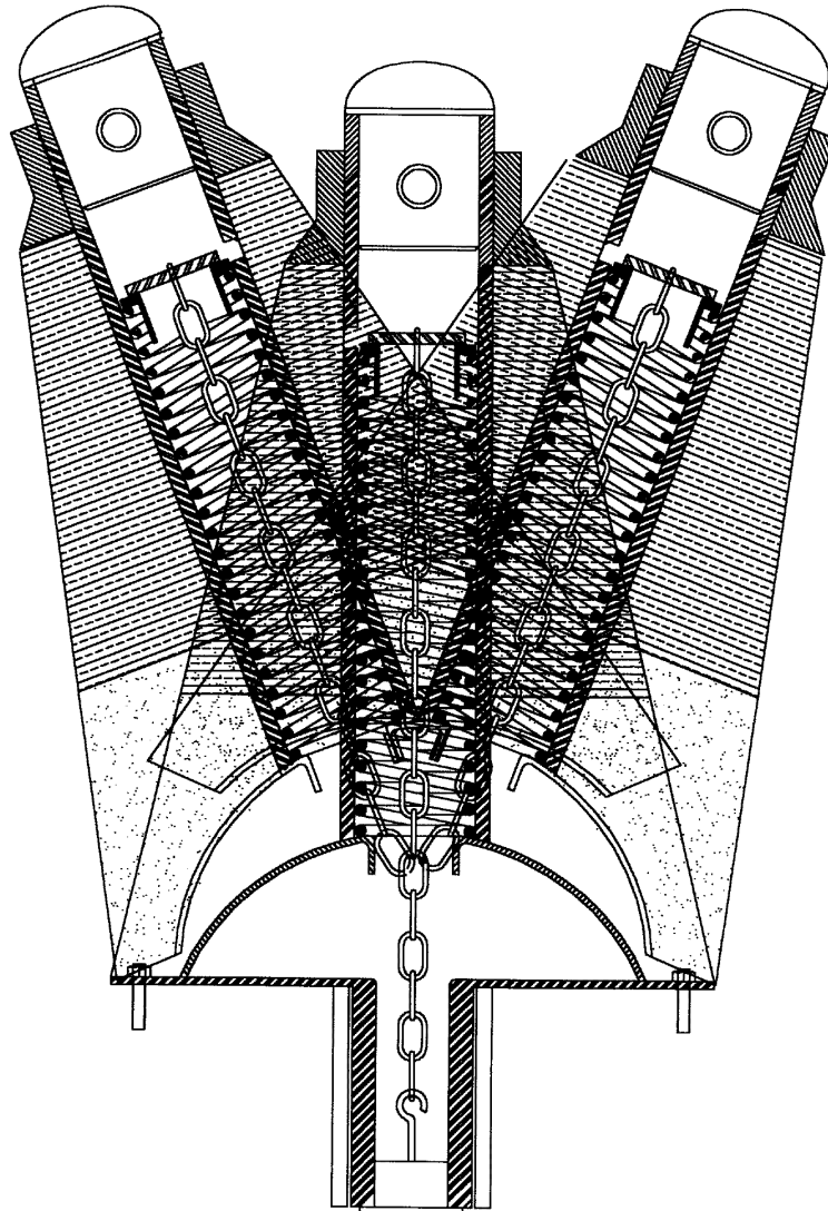
조립도-2
