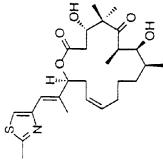
desoxyepothilone A
