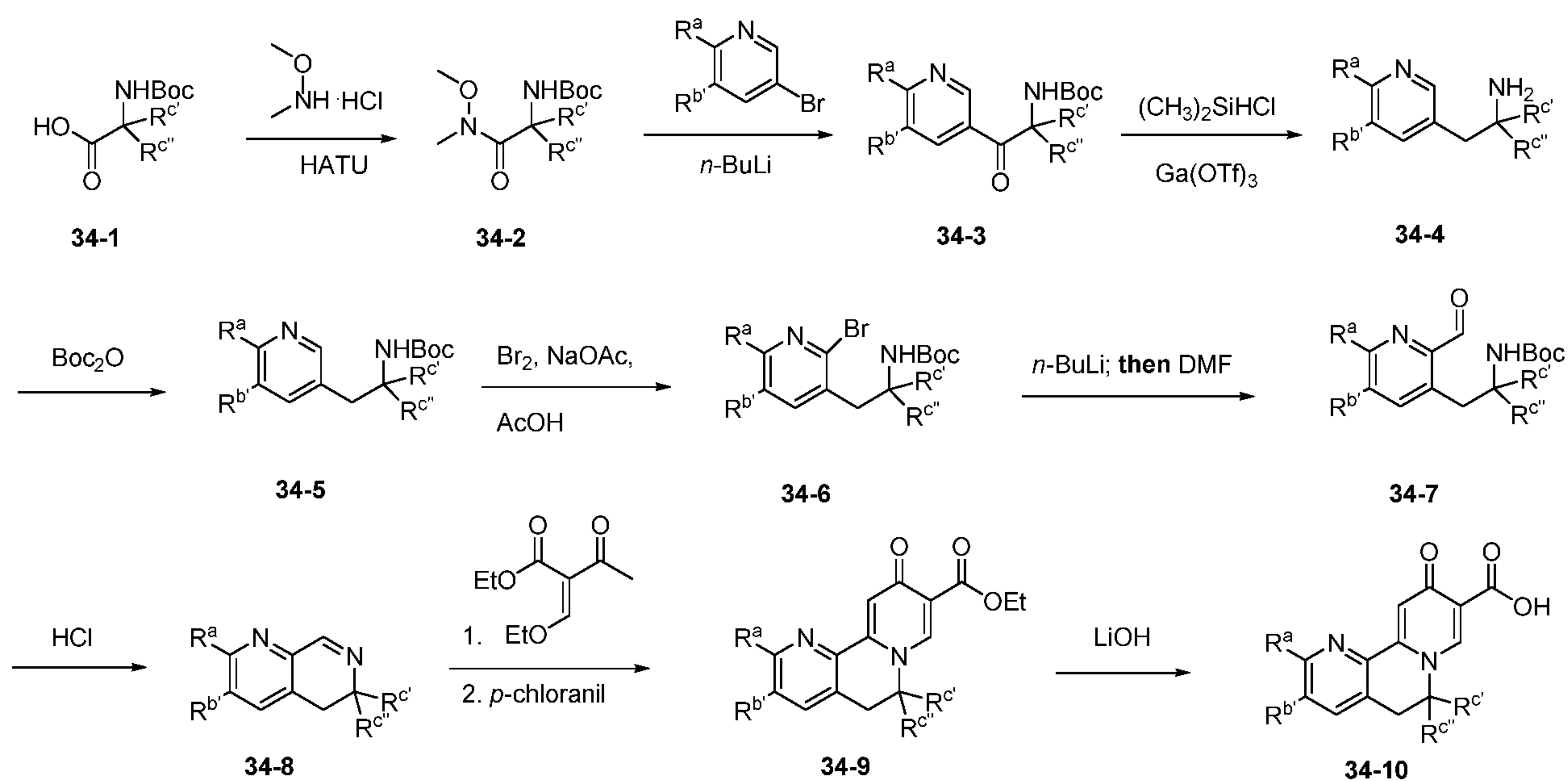
Scheme XXXIV.
