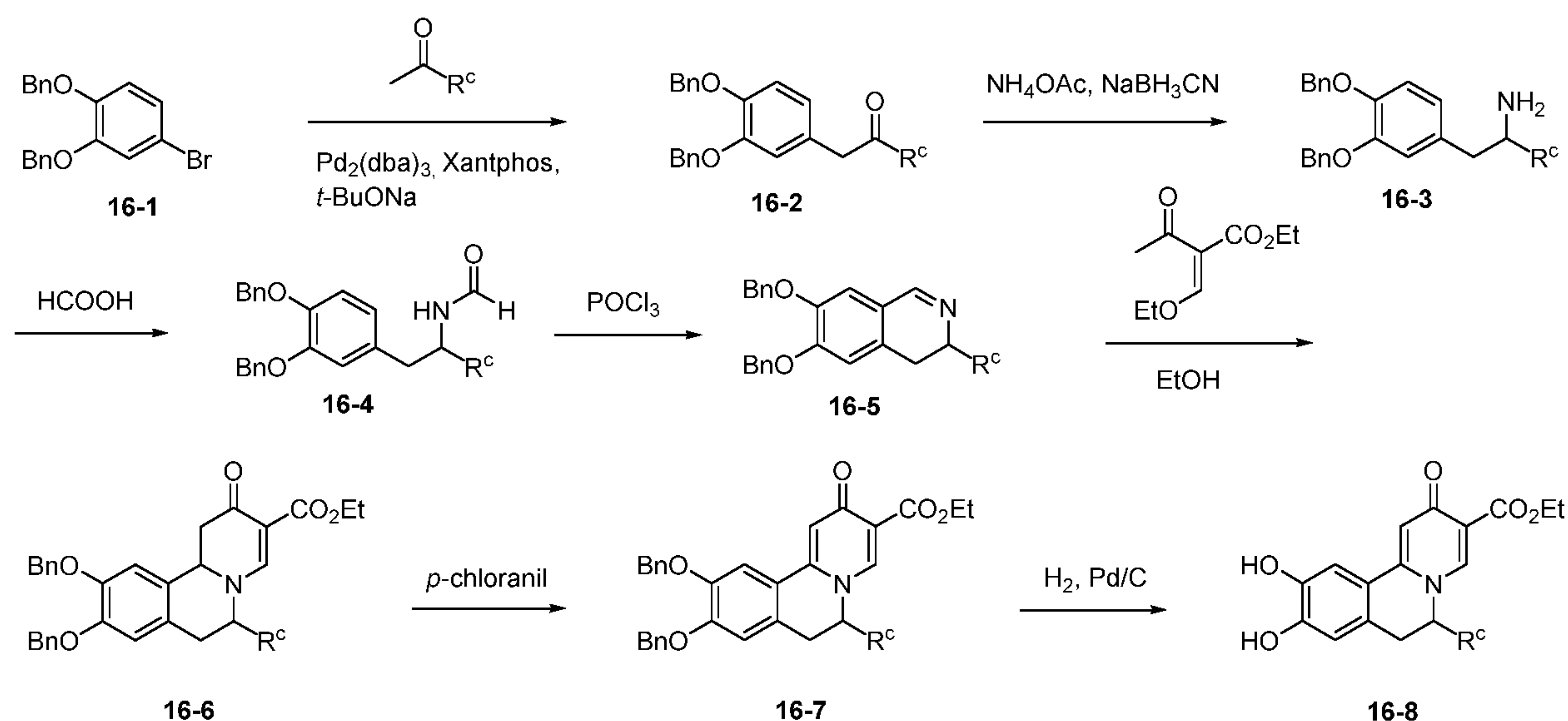
Scheme XVI.
