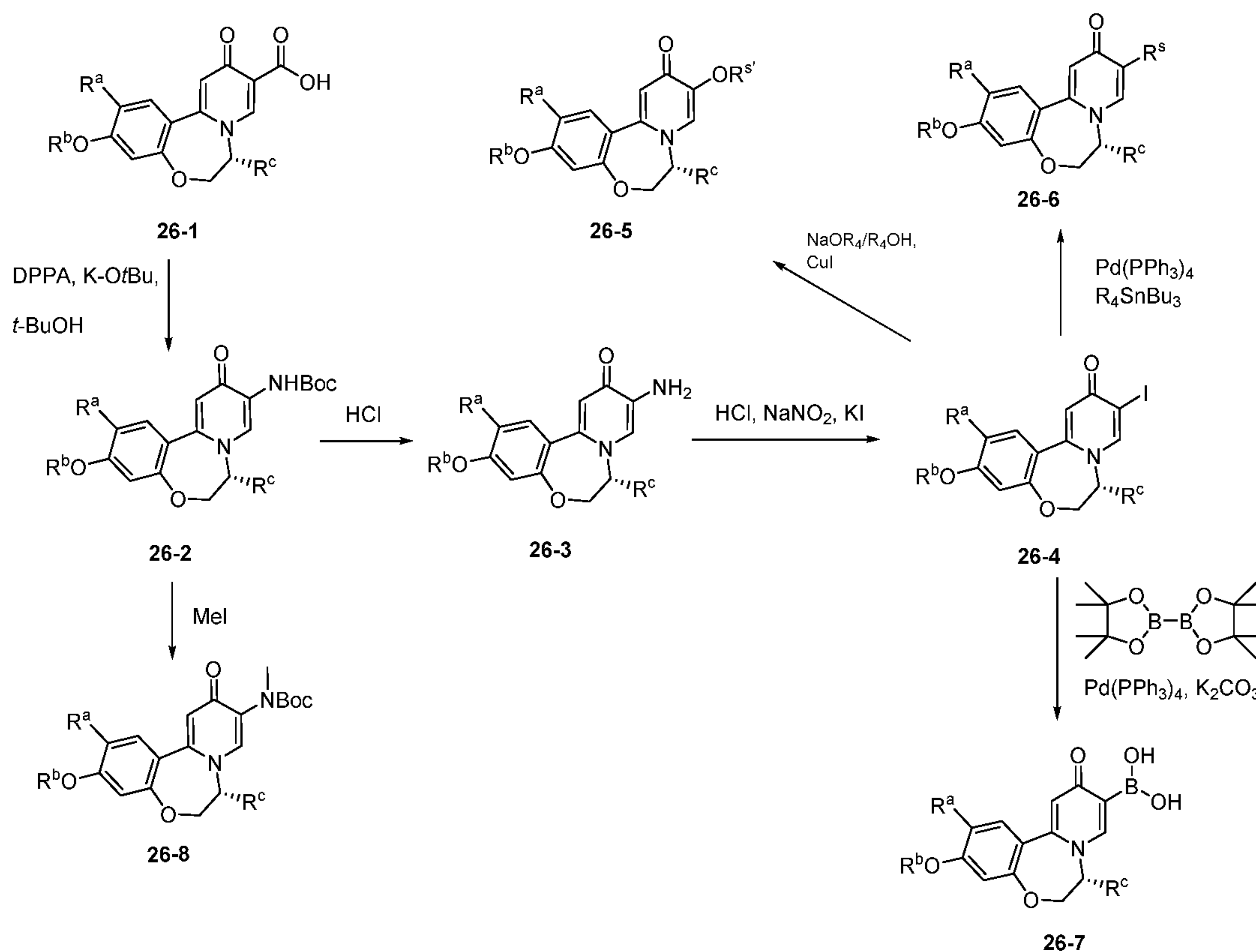
Scheme XXVI.
