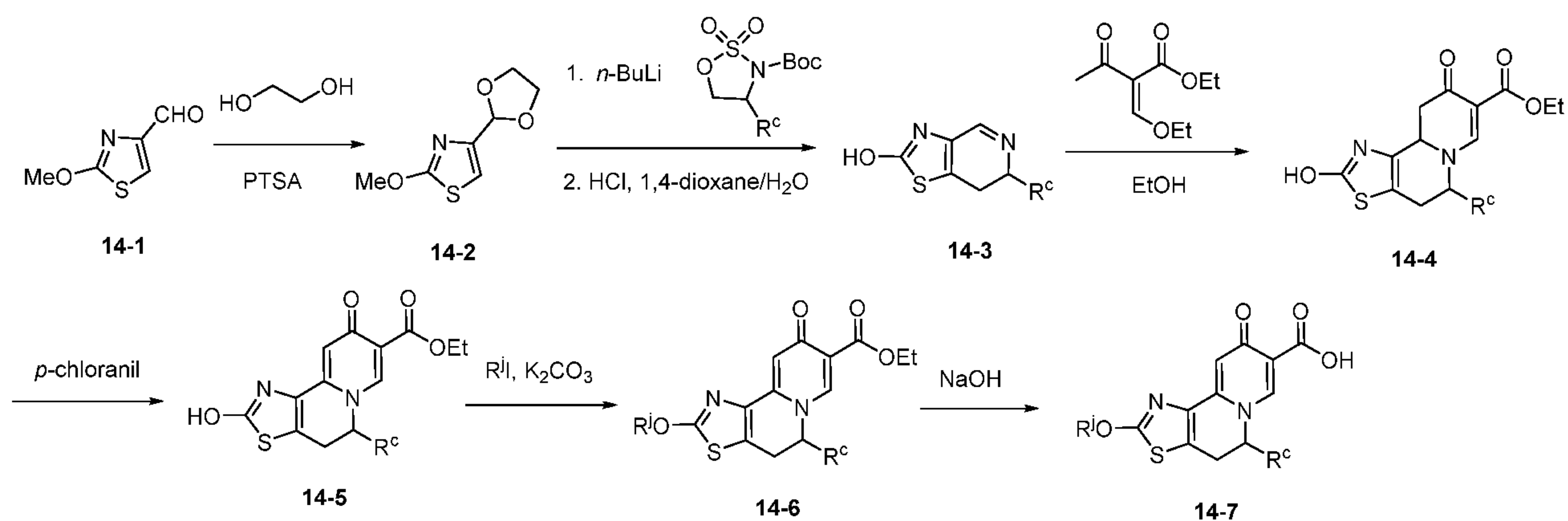
Scheme XIV.
