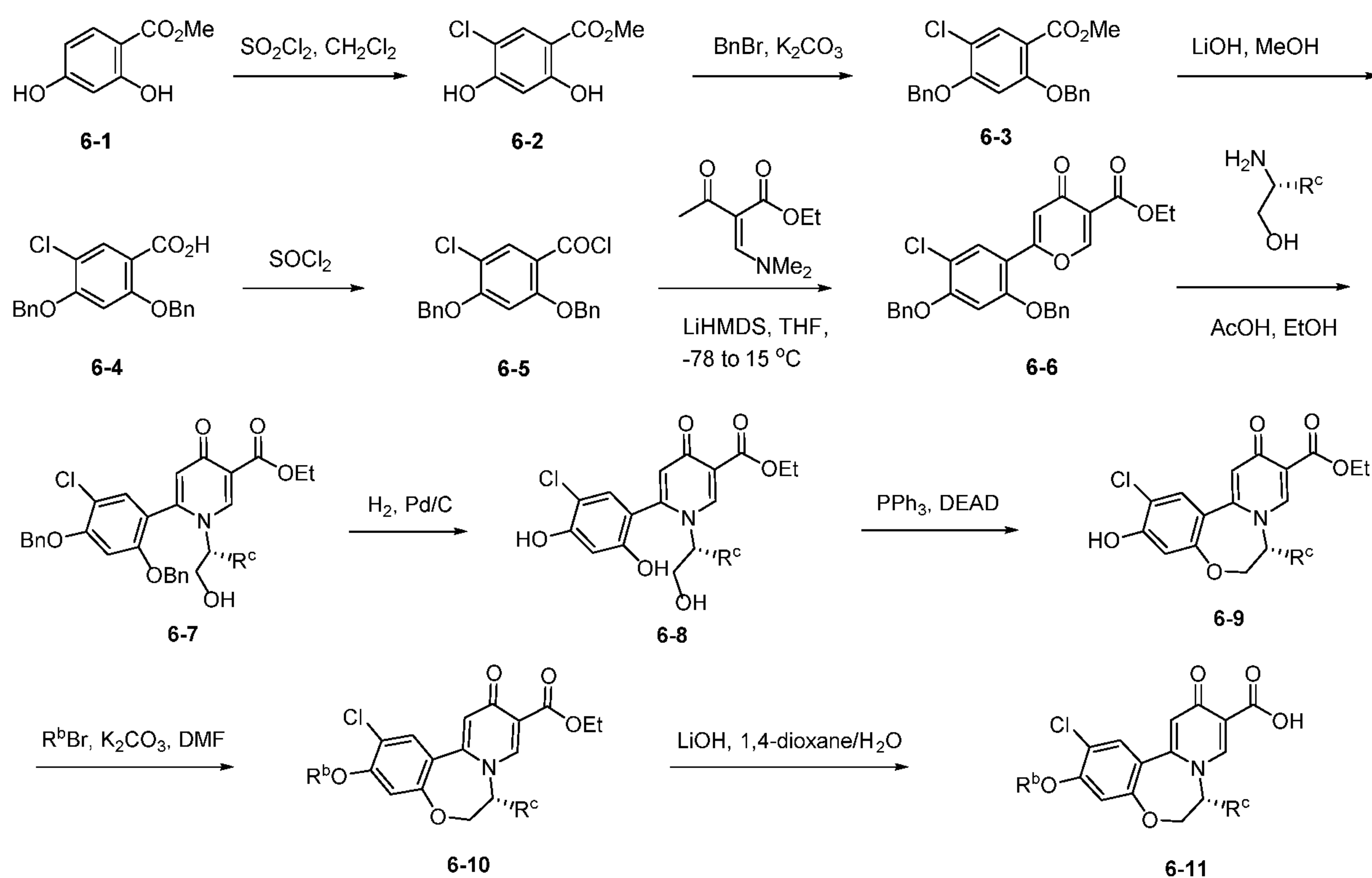
Scheme VI.
