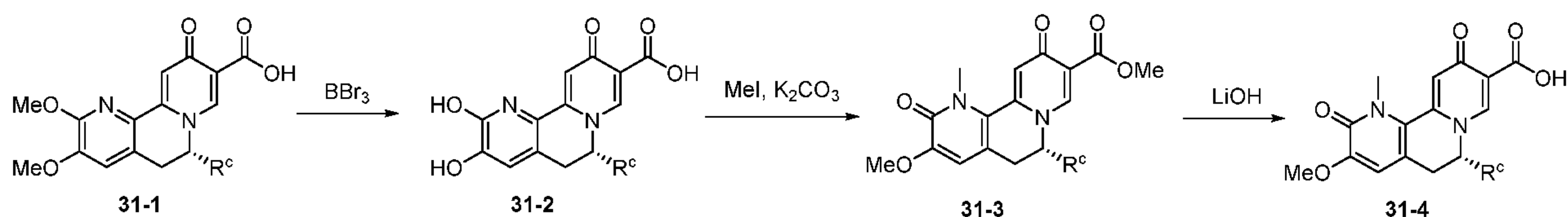
Scheme XXXI.
