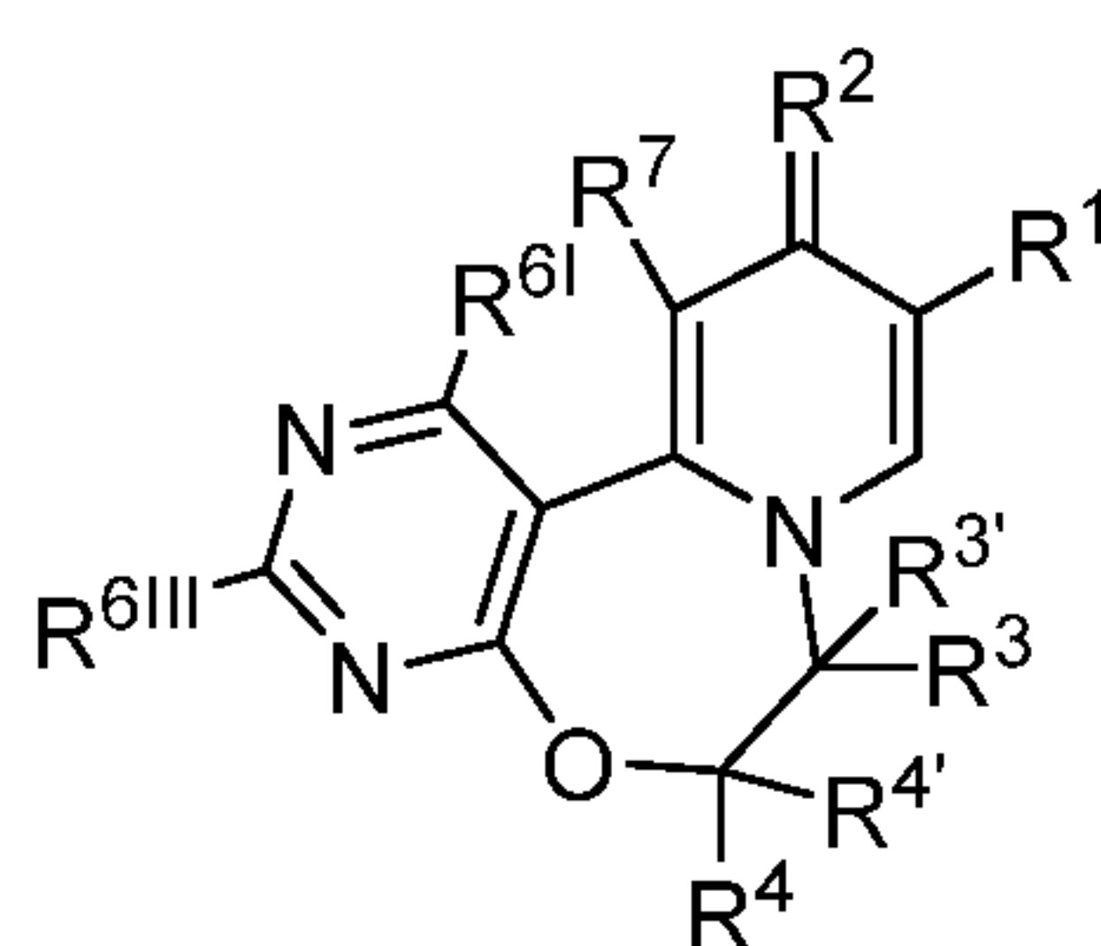
(Ip),
