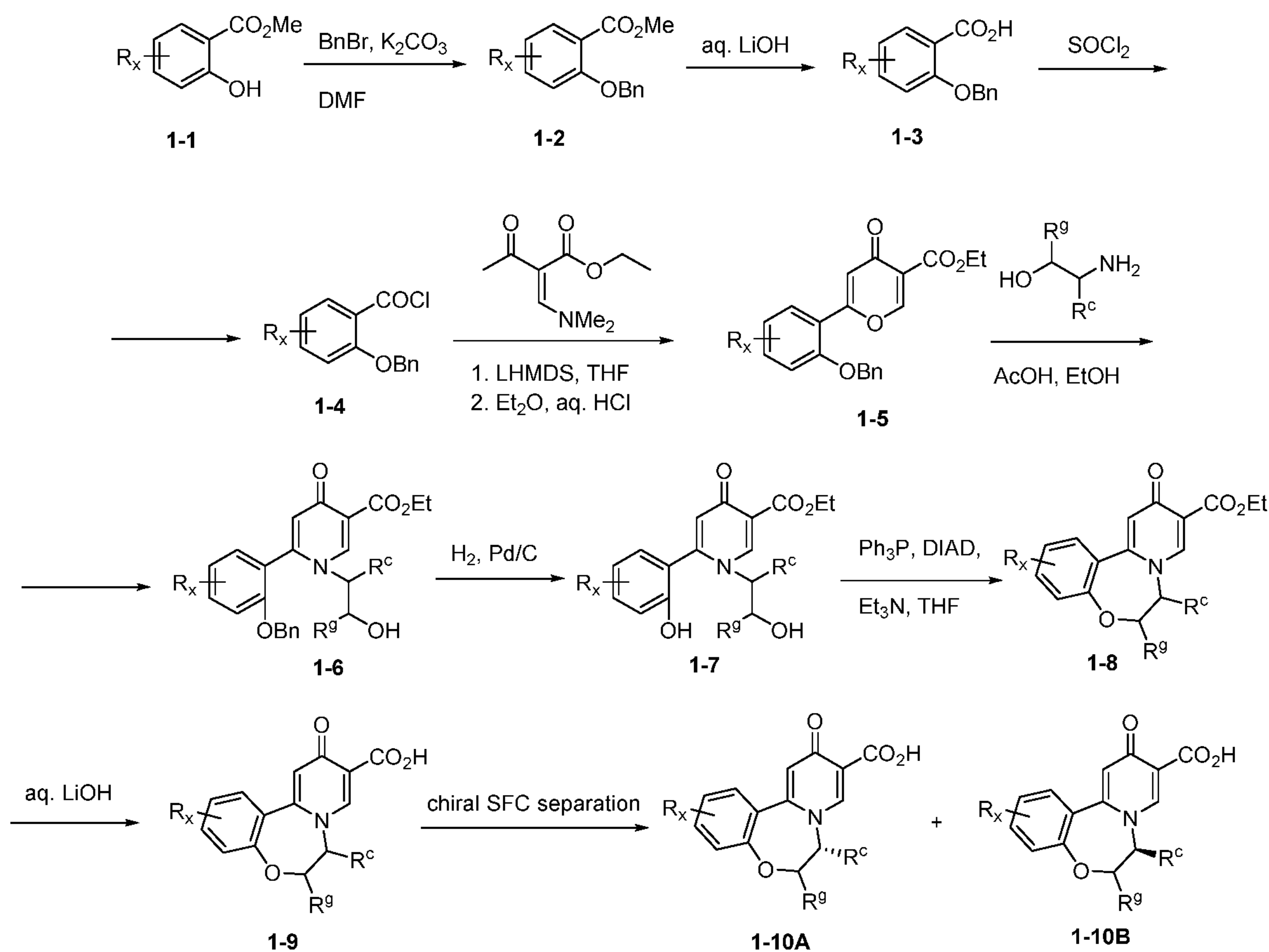
Scheme I.
