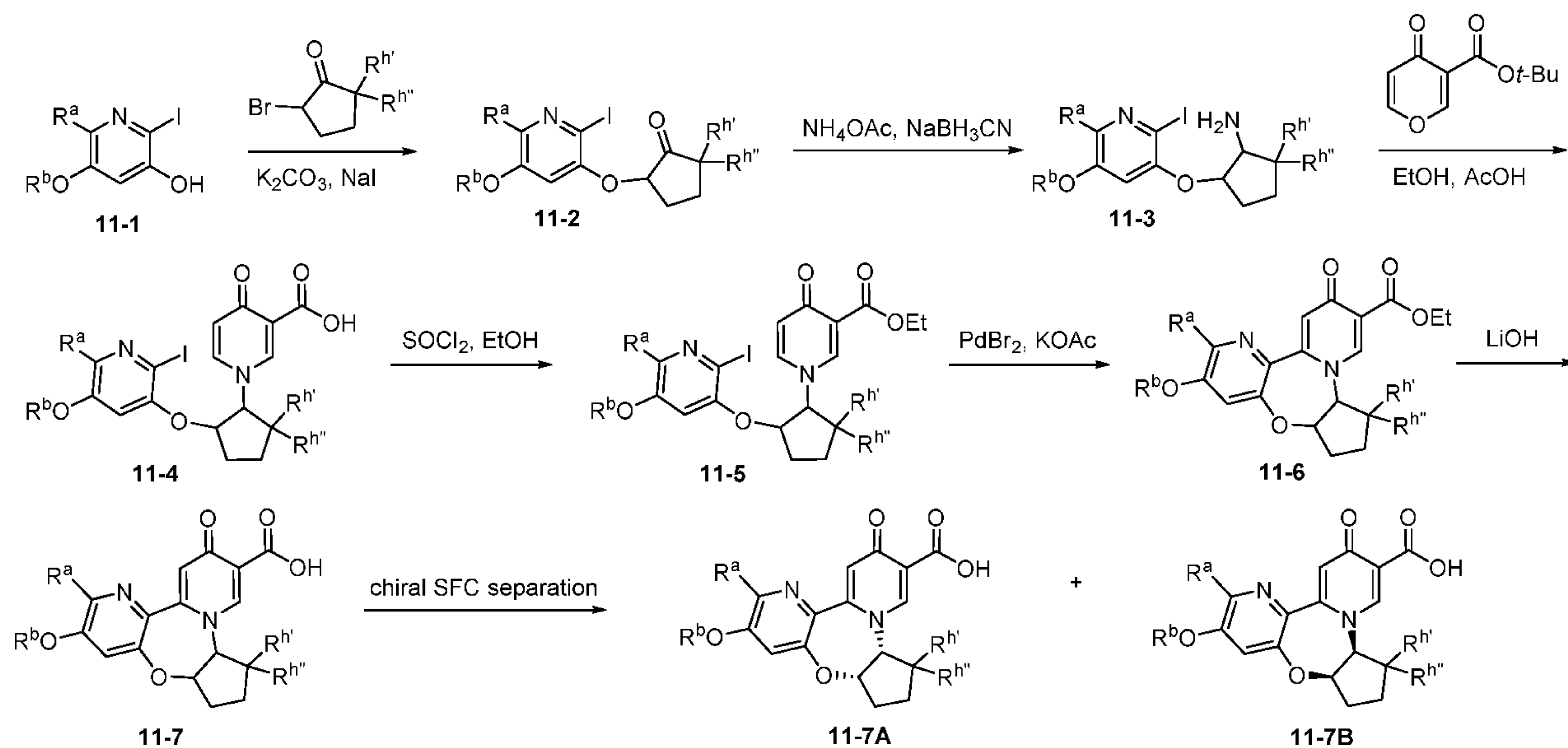
Scheme XI.
