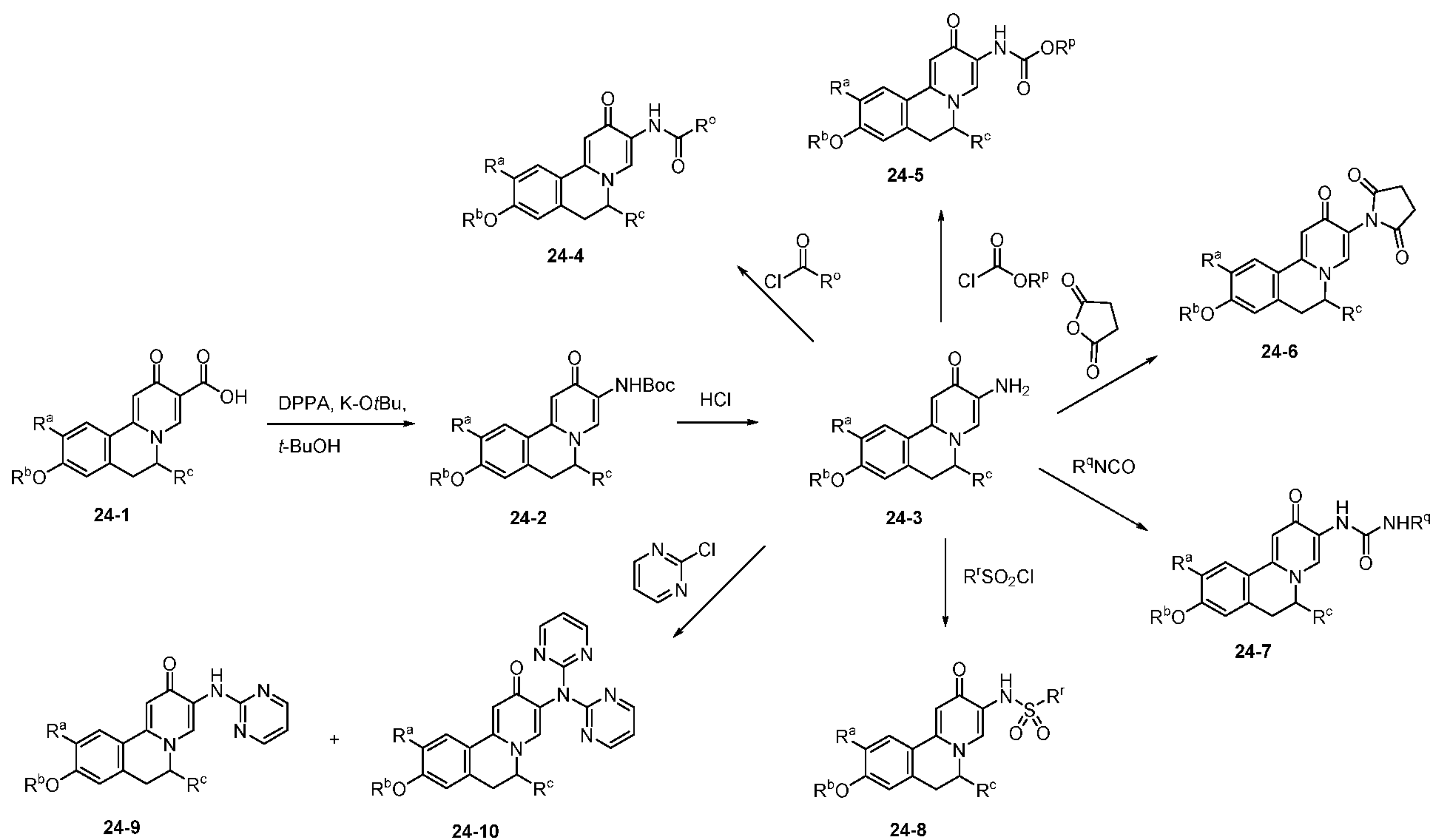
Scheme XXIV.
