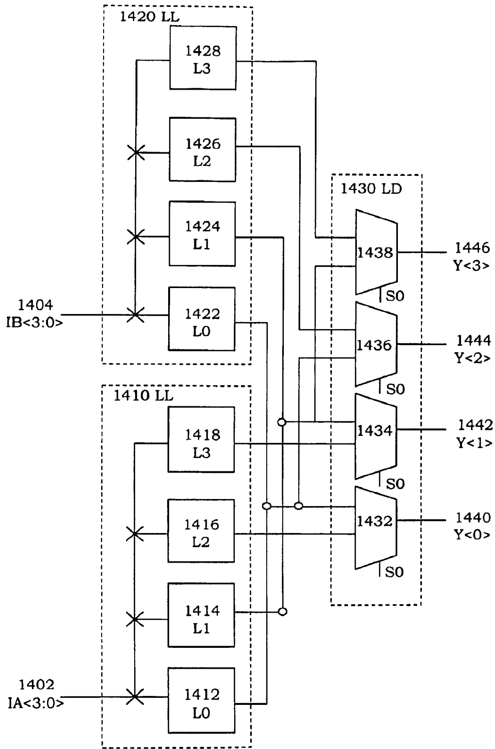
1400 4 2:1 multiplexer
