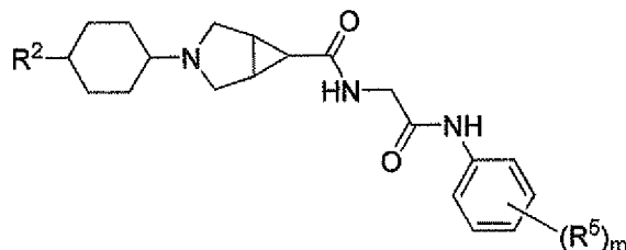
IIb
