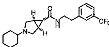
Intermediate 1e
