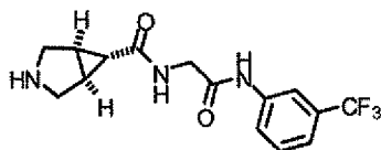
Intermediate 4e
